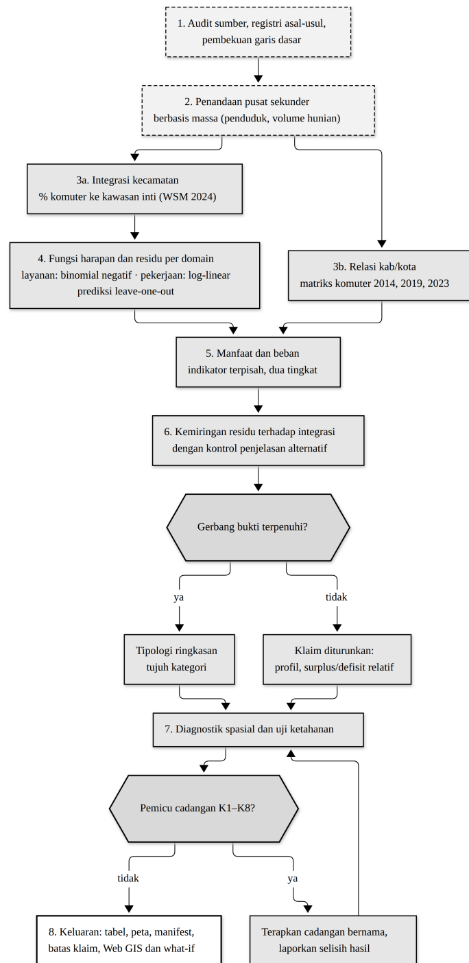
Gambar 3.2: Alur analisis dua tingkat dari audit sumber hingga keluaran. Gerbang bukti dapat menurunkan tingkat klaim, dan cadangan bernama hanya dipakai bila pemicunya terpenuhi.
