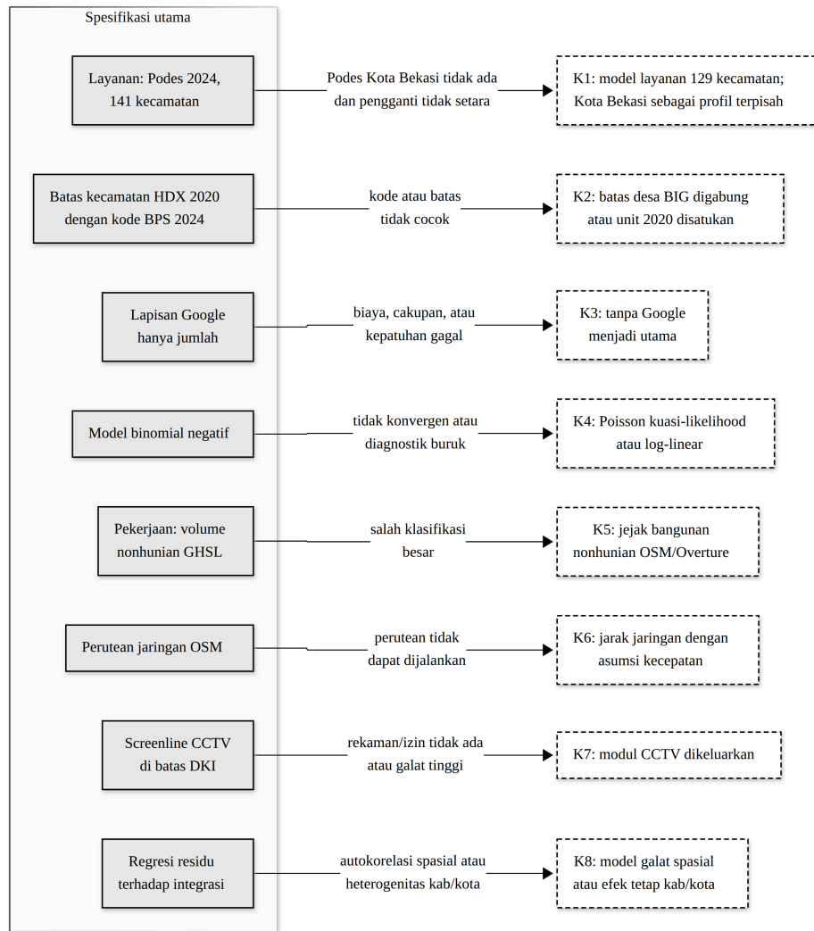
Gambar 3.1: Diagram keputusan spesifikasi utama dan cadangan bernama. Setiap cadangan hanya aktif bila pemicunya terpenuhi; selain itu rantai utama dipertahankan.
