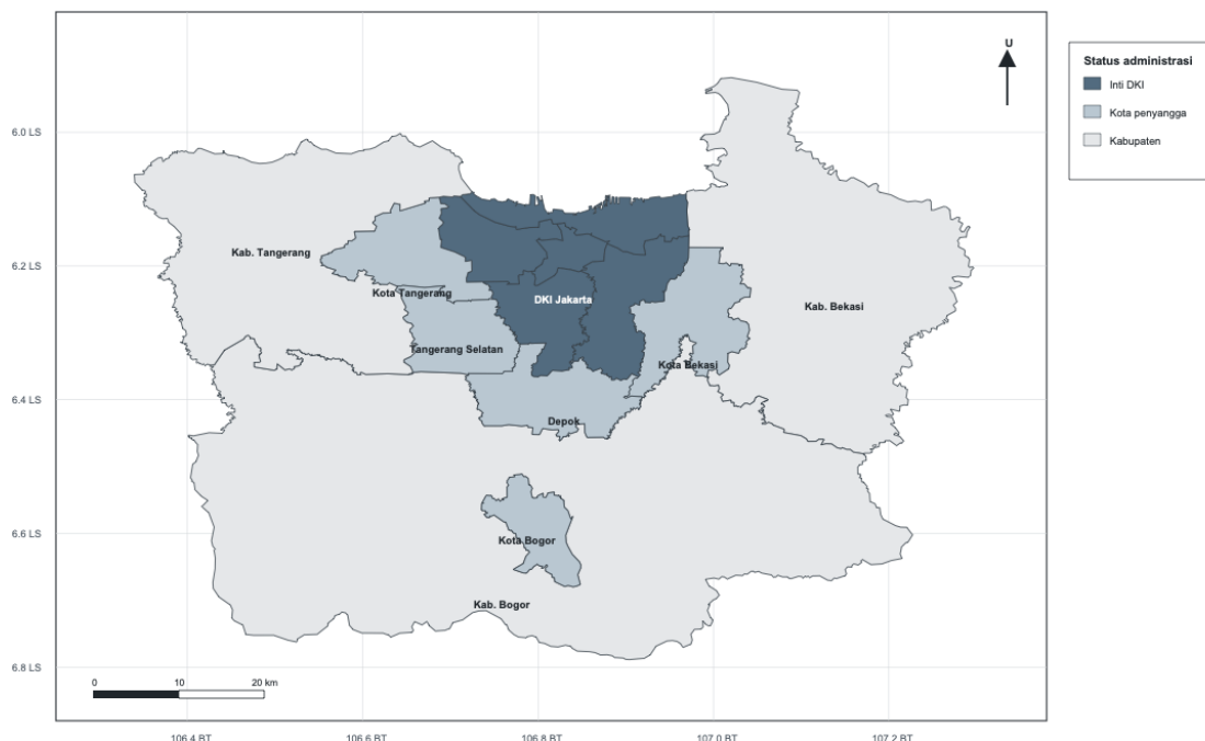
Gambar 4.1: Batas dan status administratif wilayah penelitian (gambar sementara). Sumber geometri: geoBoundaries gbOpen Indonesia ADM2, build 2023 dengan batas tahun 2020 (William & Mary GeoLab 2023). Kelas membedakan inti DKI, kota, dan kabupaten untuk pelaporan; kelas tersebut bukan ukuran morfologi atau kematangan pusat. Peta final memakai proyeksi UTM 48S dan memuat kabupaten tetangga, termasuk Cianjur, sebagai konteks.
