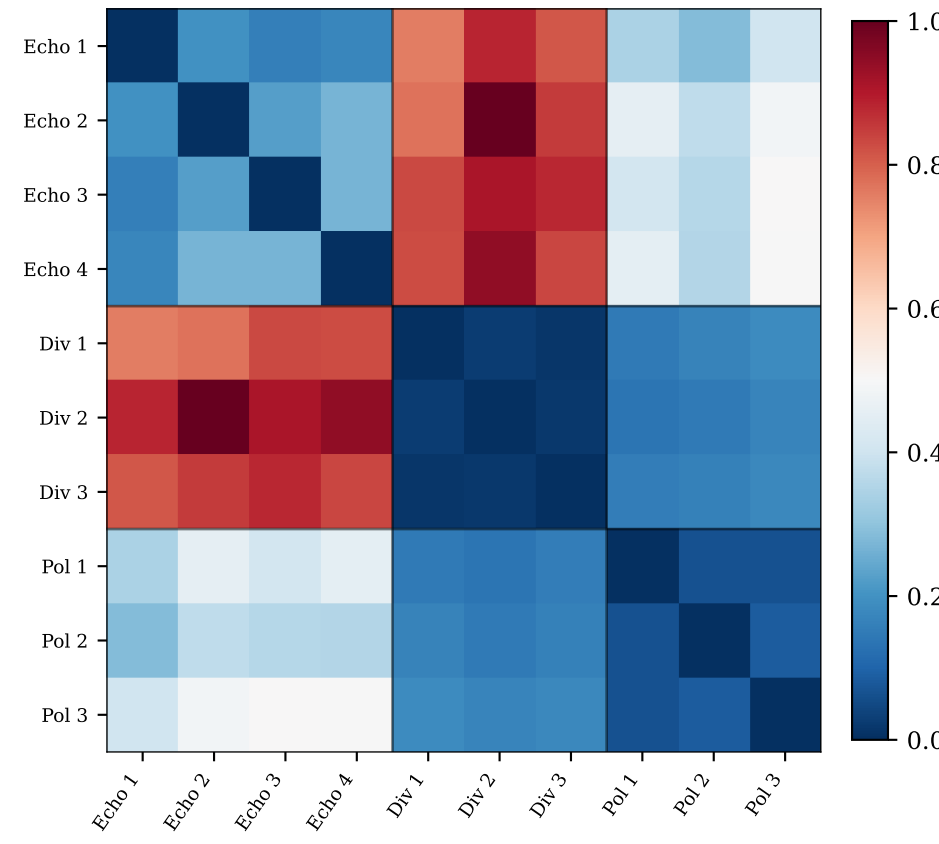
KL Divergence
