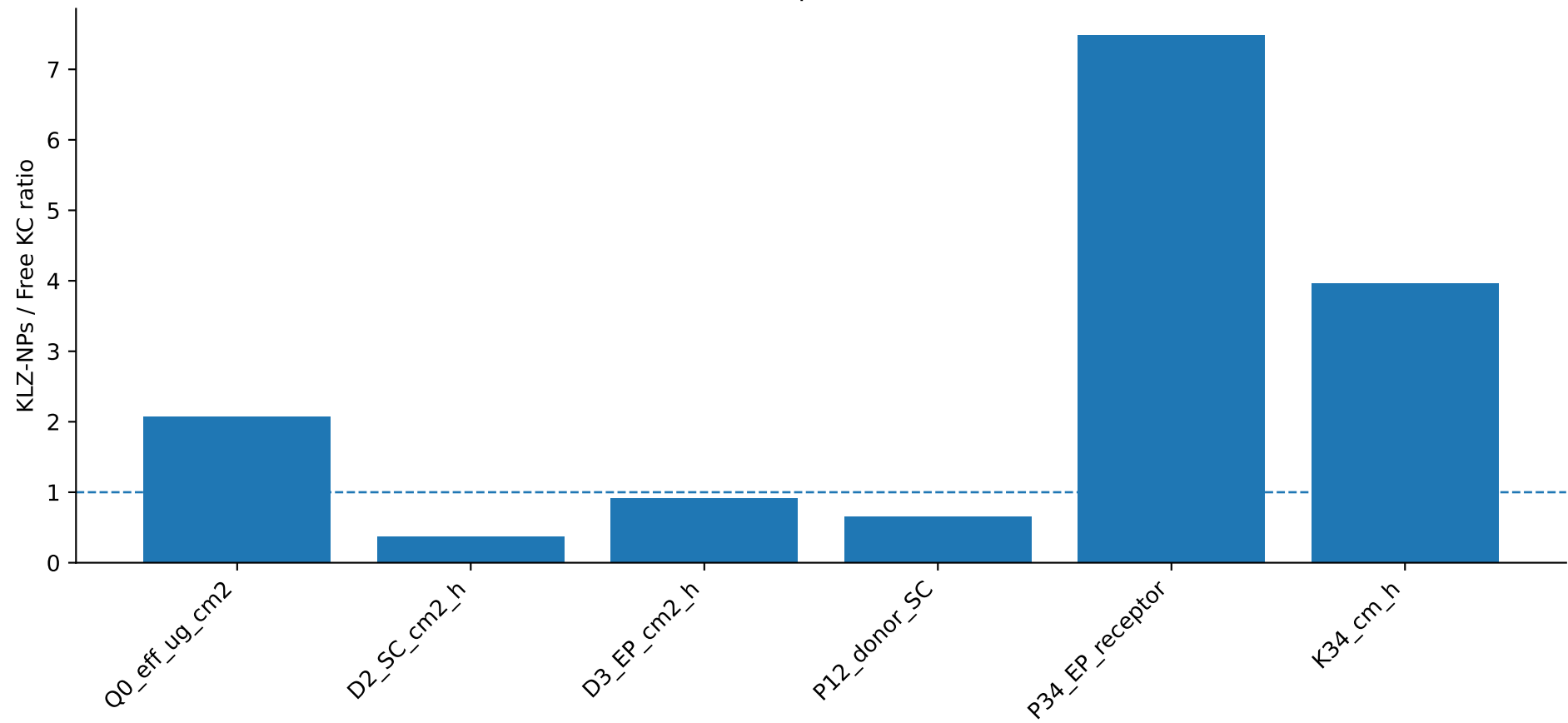
Case 1 fitted parameter ratios
