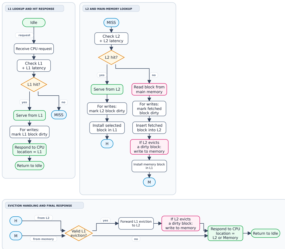
شکل ۱: ماشین حالت پردازش درخواست در معماری پایه 11-12
