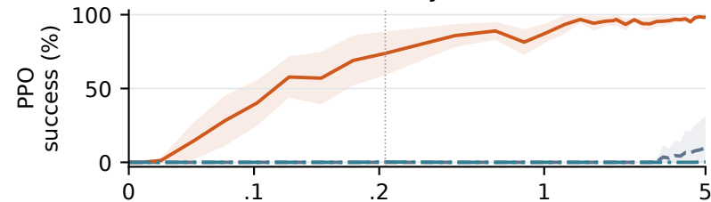
DoorKey-8x8
