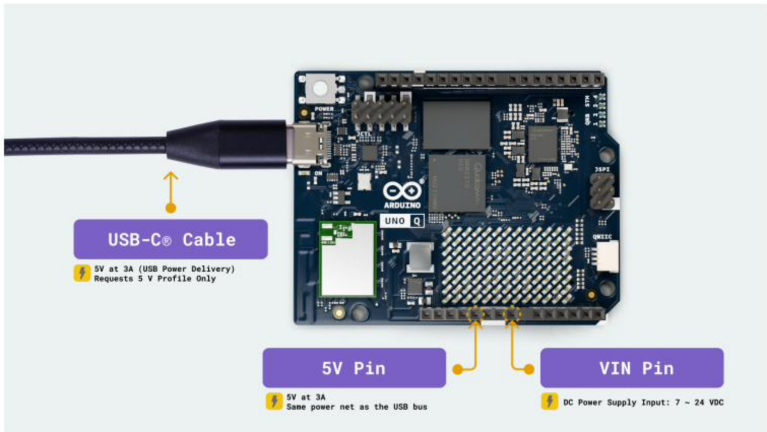
UNO Q Input Methods
