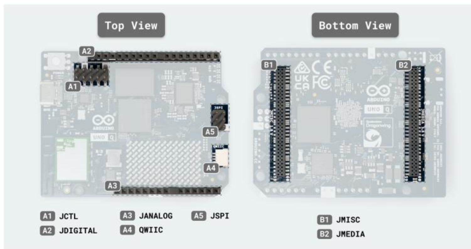
UNO Q Peripherals
