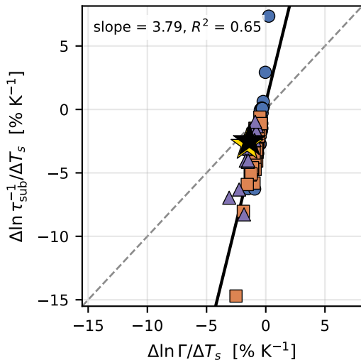
(d) Offset universality
