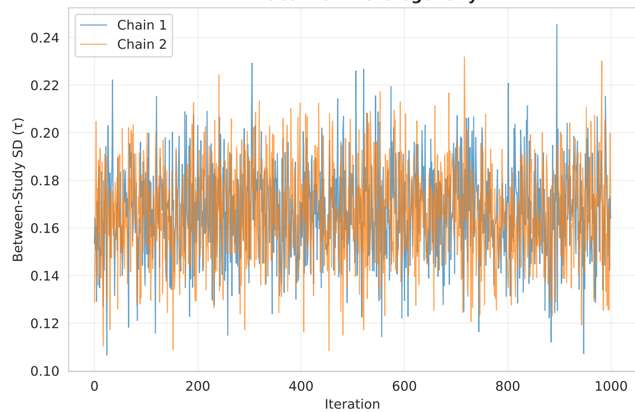
D. Posterior Distribution: \tau
