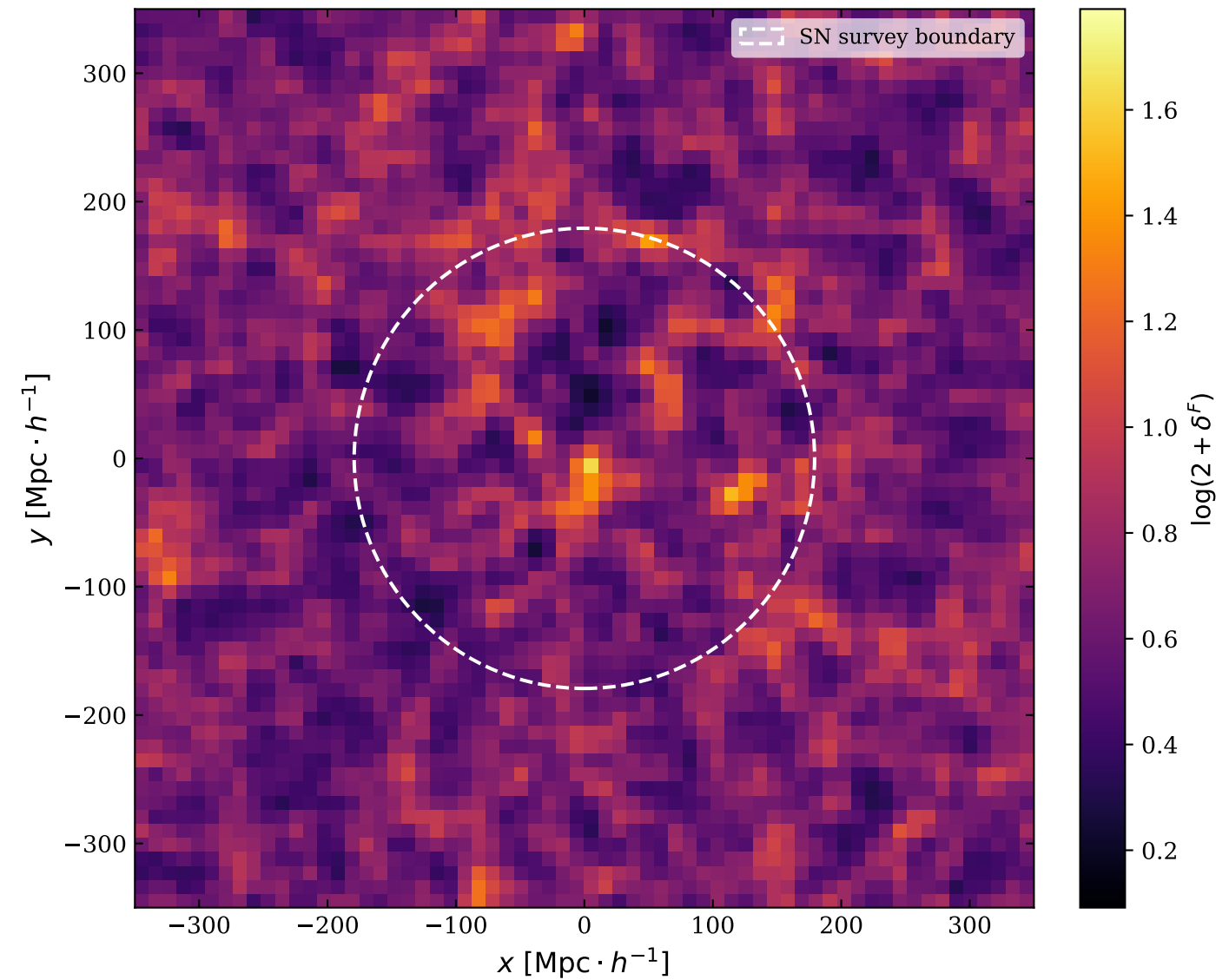
Mean posterior \langle \delta^F \rangle
