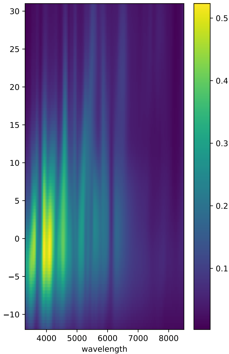
SALT3
