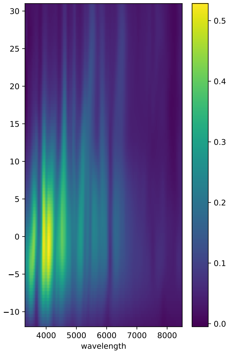
SALT2.4
