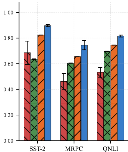
GPT-2
