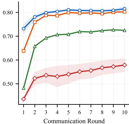
GPT-2
