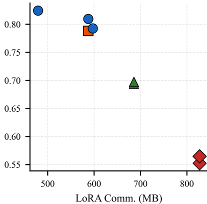
GPT-2
