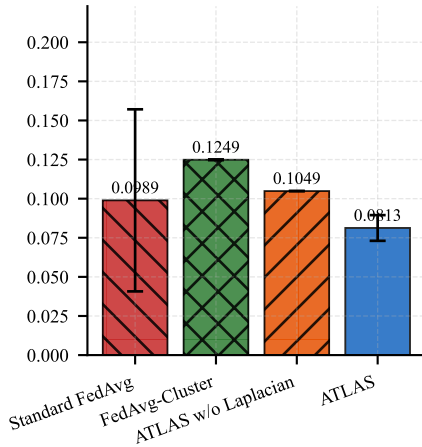
GPT-2
