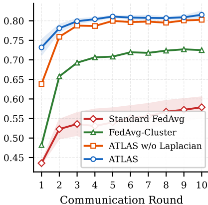
GPT-2
