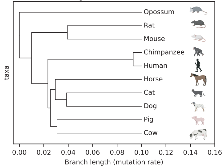
(D) Using \alpha -MaxGeomHash ( \alpha=0.45 )
