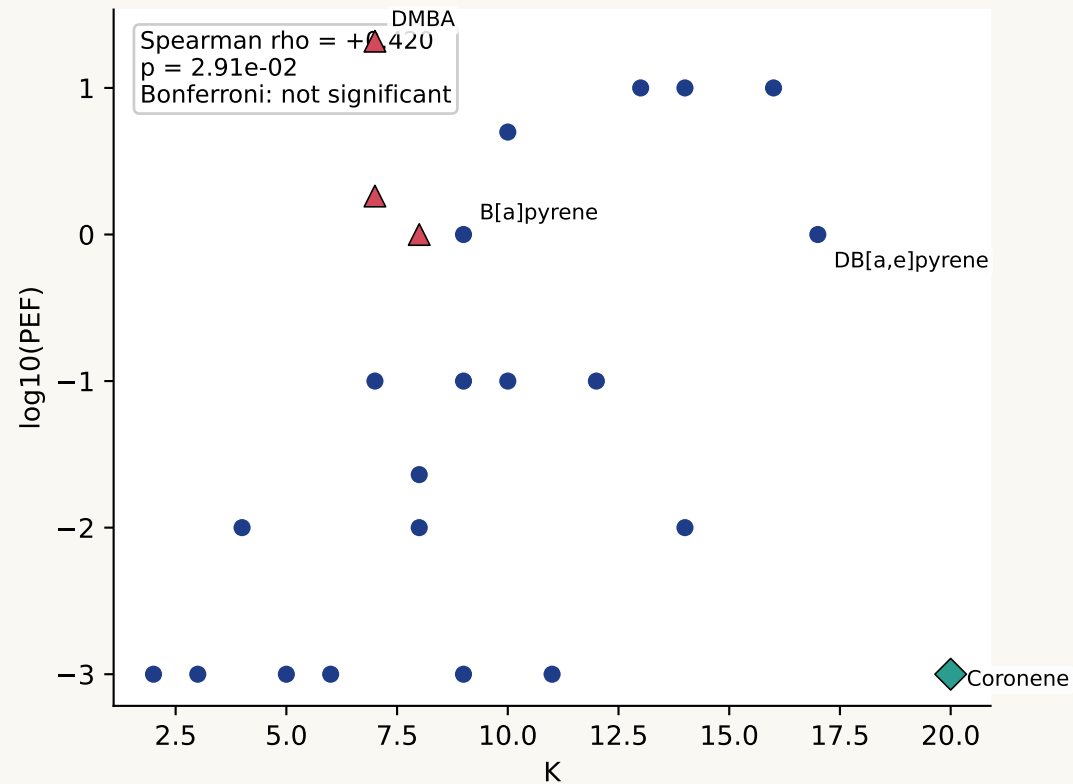
A. Kekule Count Alone
