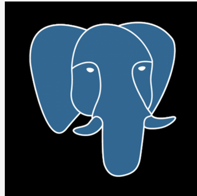
PostgreSQL
