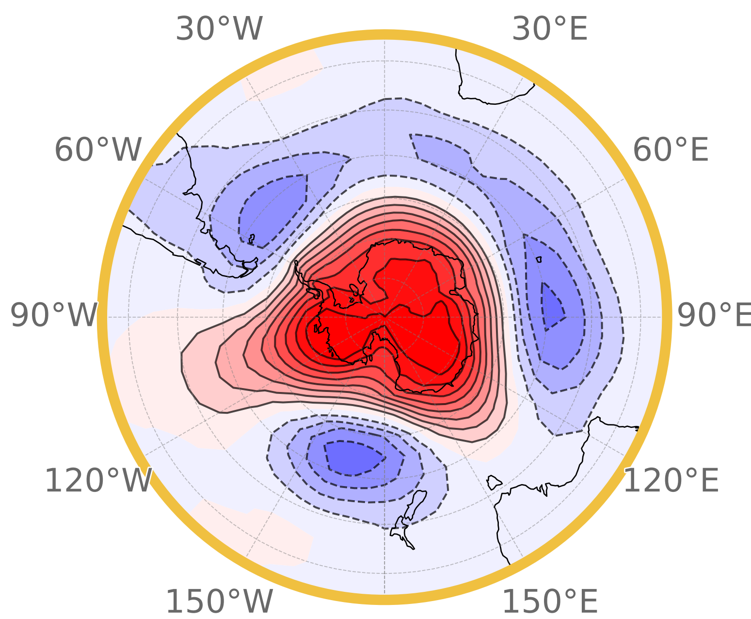
(a) MAM EOF 1 reference
