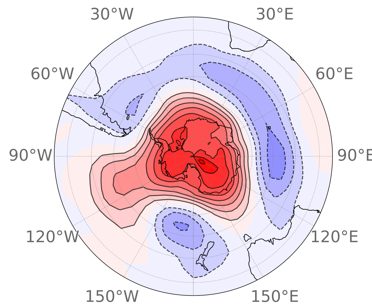
(d) MAM Cluster 3 26 events (20.2%)
