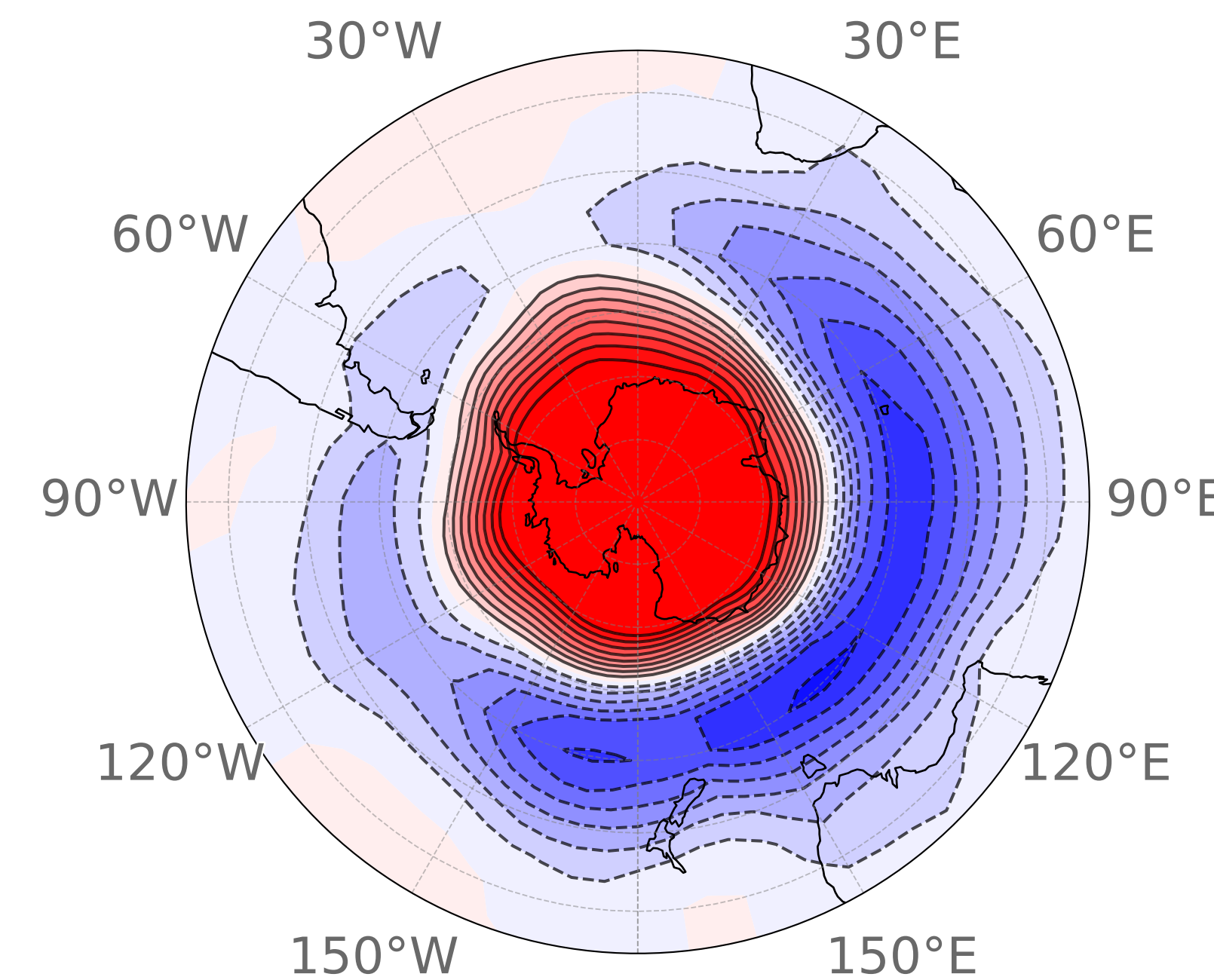
(d) SON Cluster 3 20 events (15.5%)
