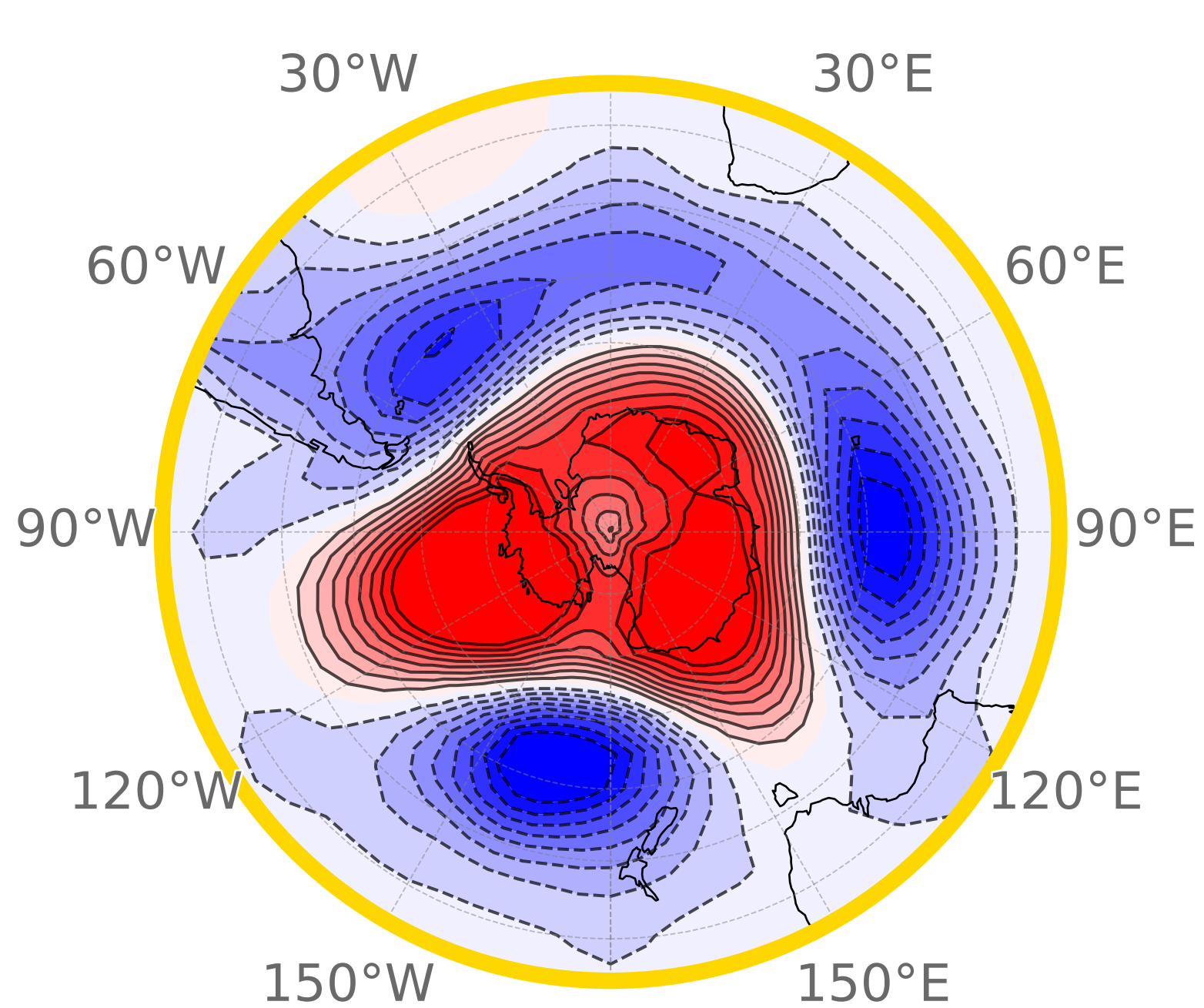
(f) MAM EOF 1 reference
