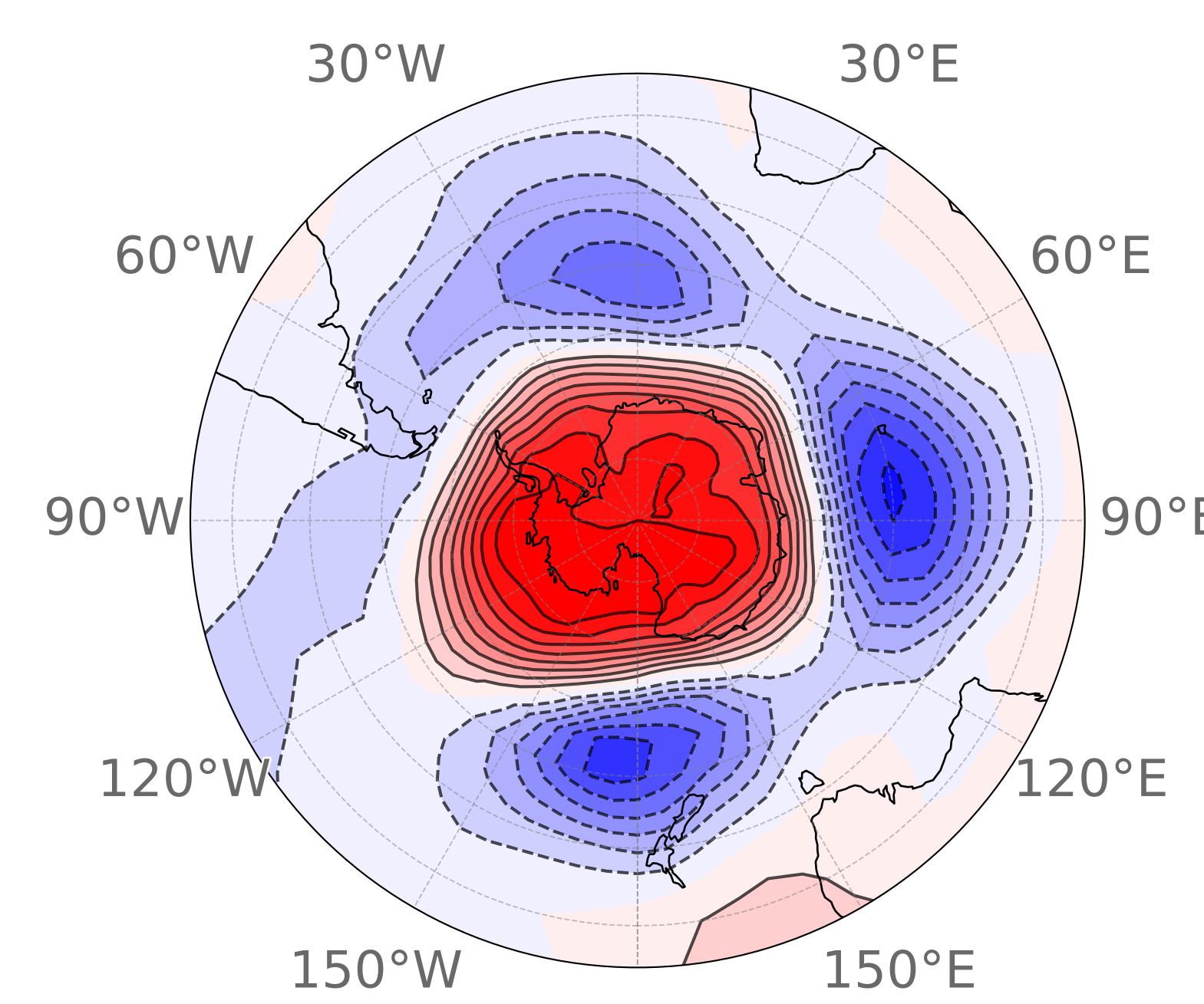
(d) DJF Cluster 3 20 events (15.5%)
