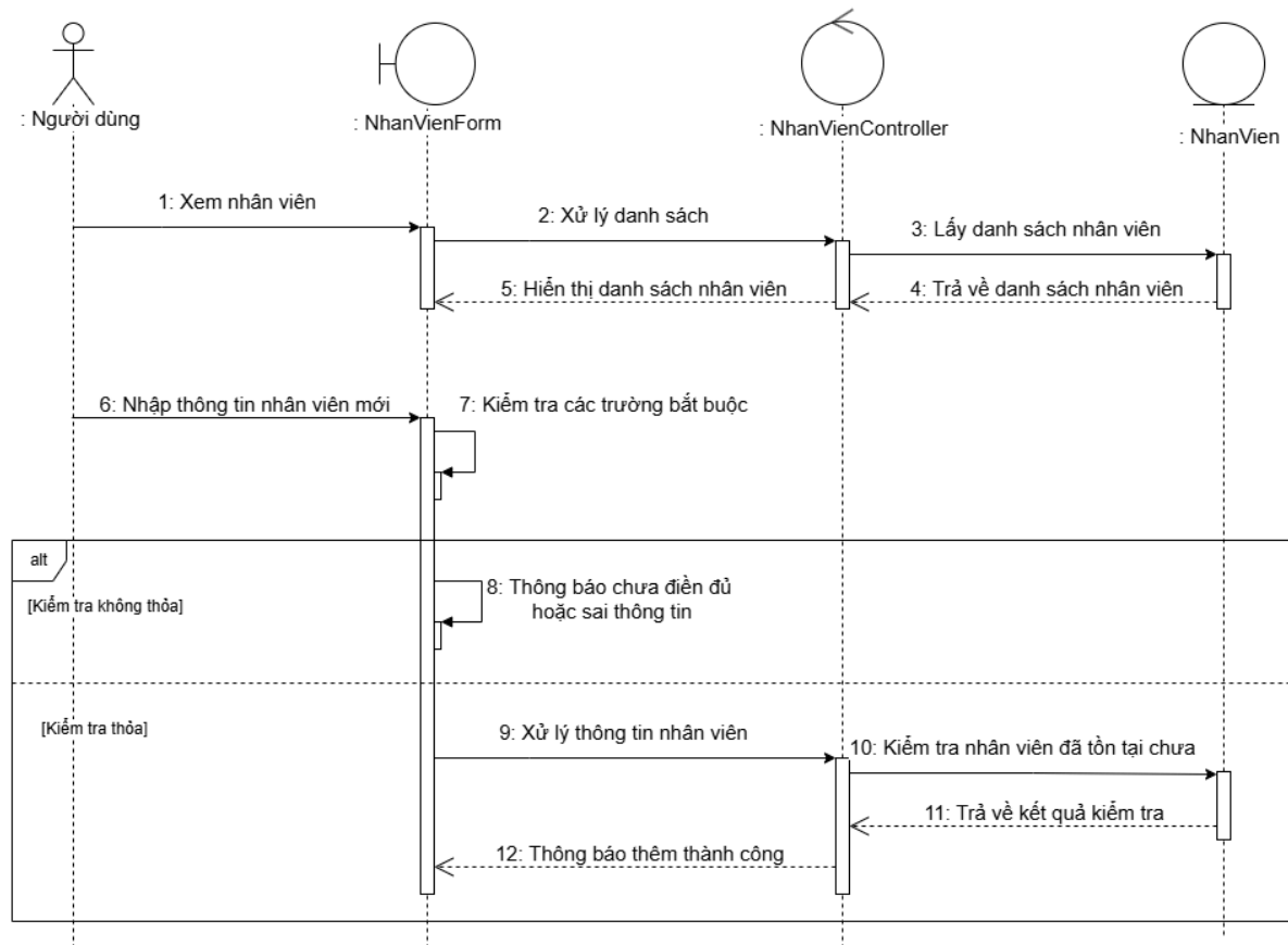
Hình 28-1. Sơ đồ tuần tự “Thêm nhân viên” trong “Quản lý nhân viên”
