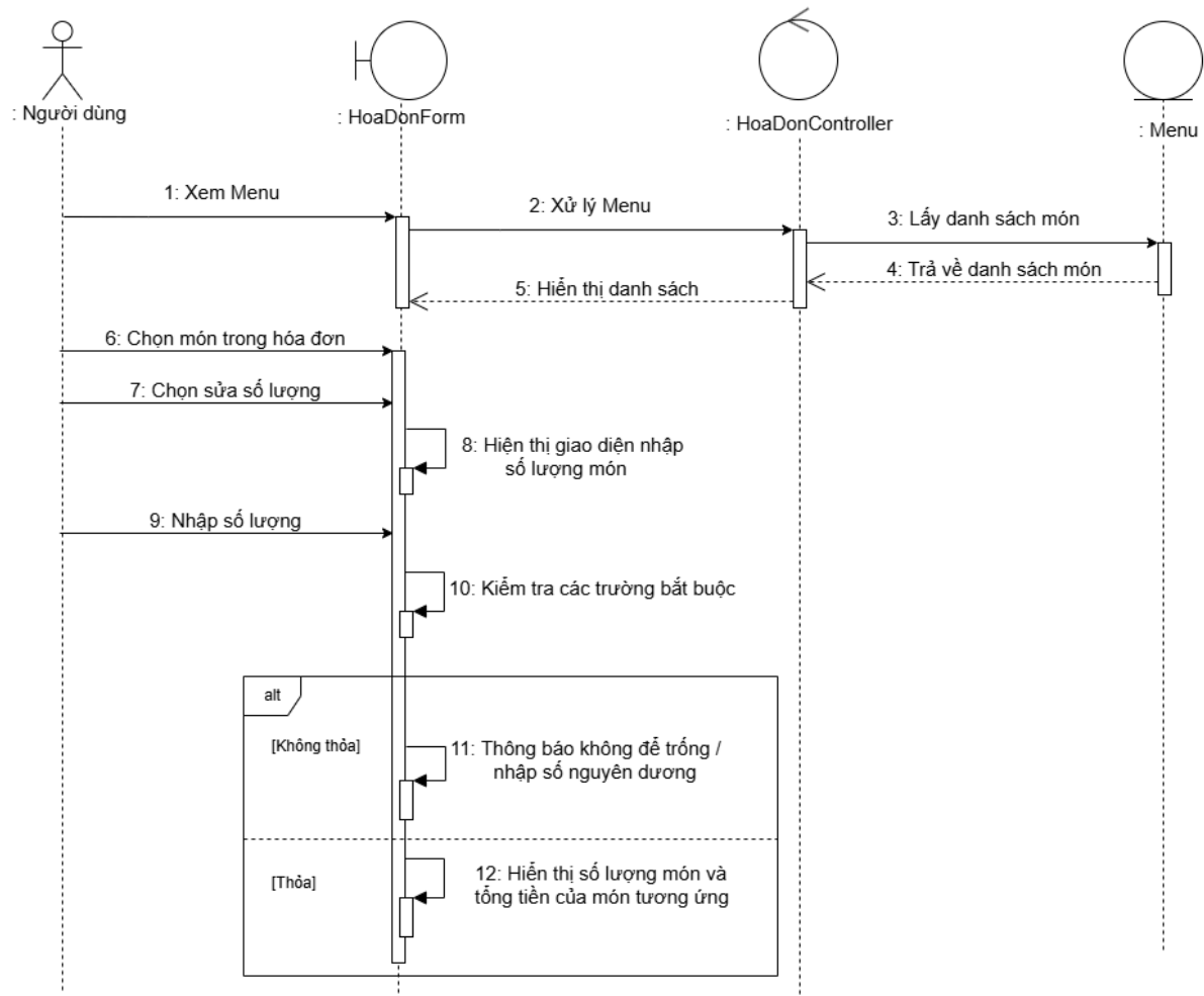
Hình 31-3. Sơ đồ tuần tự “Sửa số lượng món” trong “Tạo hóa đơn”
