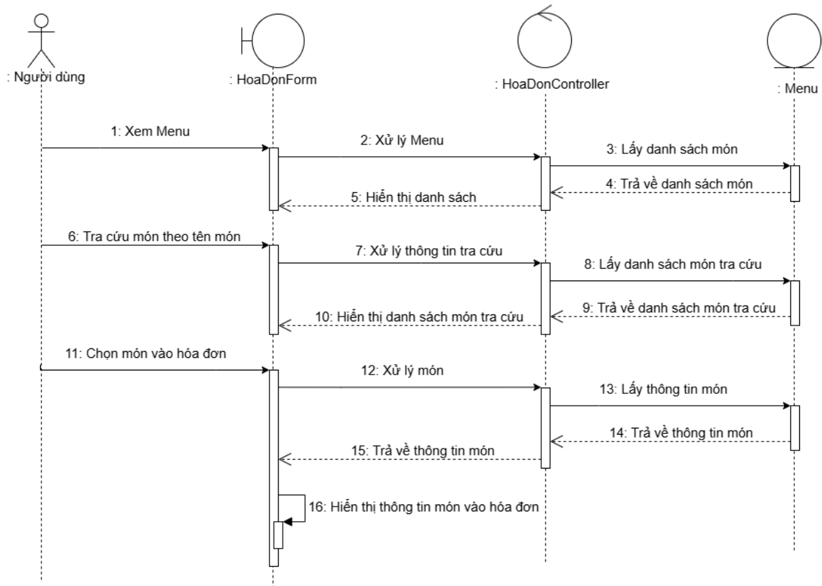
Hình 31-1. Sơ đồ tuần tự “Chọn món” trong “Tạo hóa đơn”
