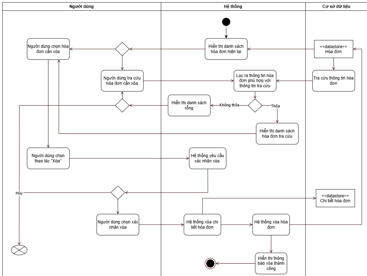
Hình 19. Activity Diagram “Xóa hóa đơn”
