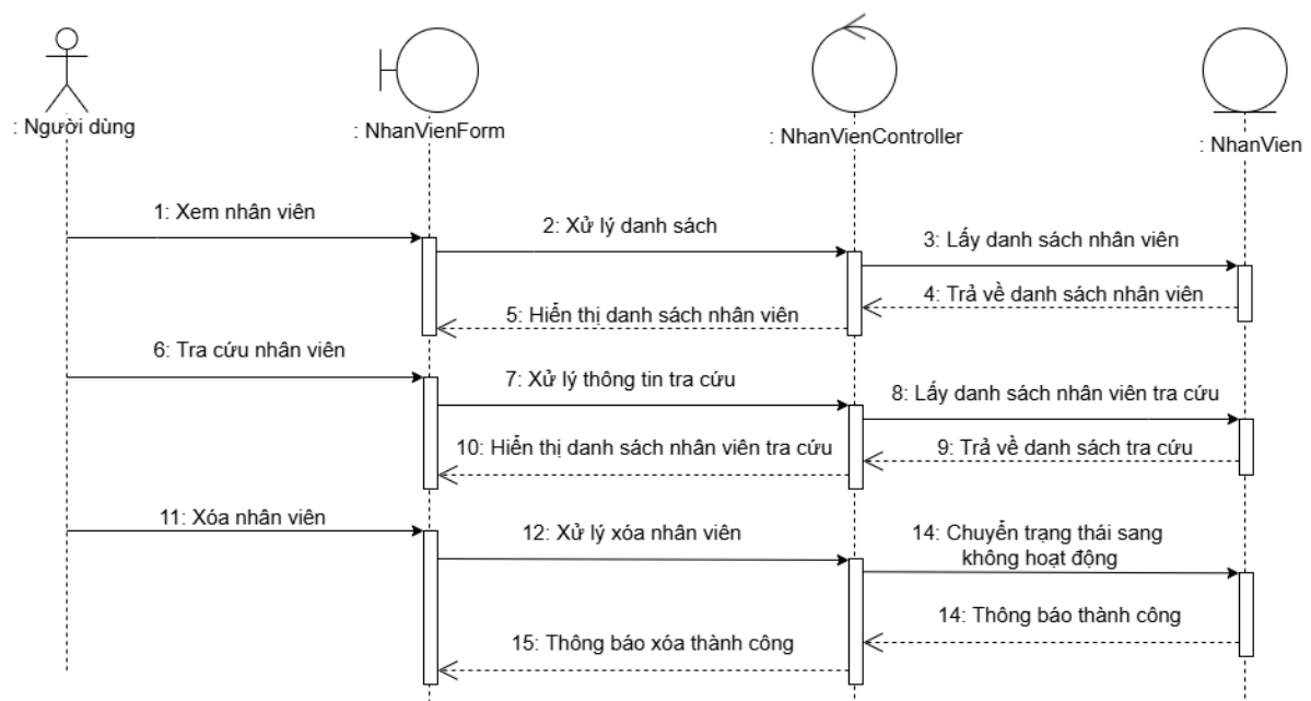
Hình 28-3. Sơ đồ tuần tự “Xóa nhân viên” trong “Quản lý nhân viên”
