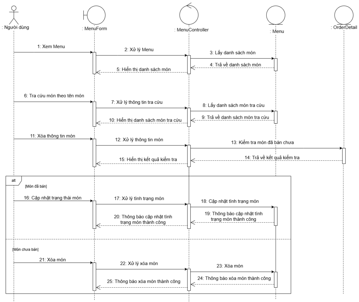
Hình 27-3. Sơ đồ tuần tự “Xóa món” trong “Quản lý Menu”
