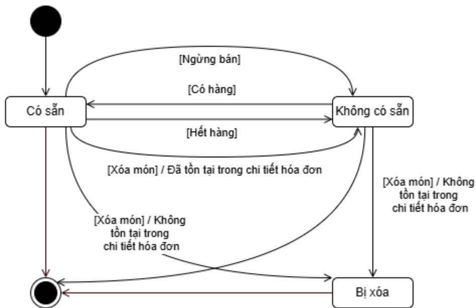
Hình 34. Sơ đồ trạng thái cho đối tượng MENUITEM
