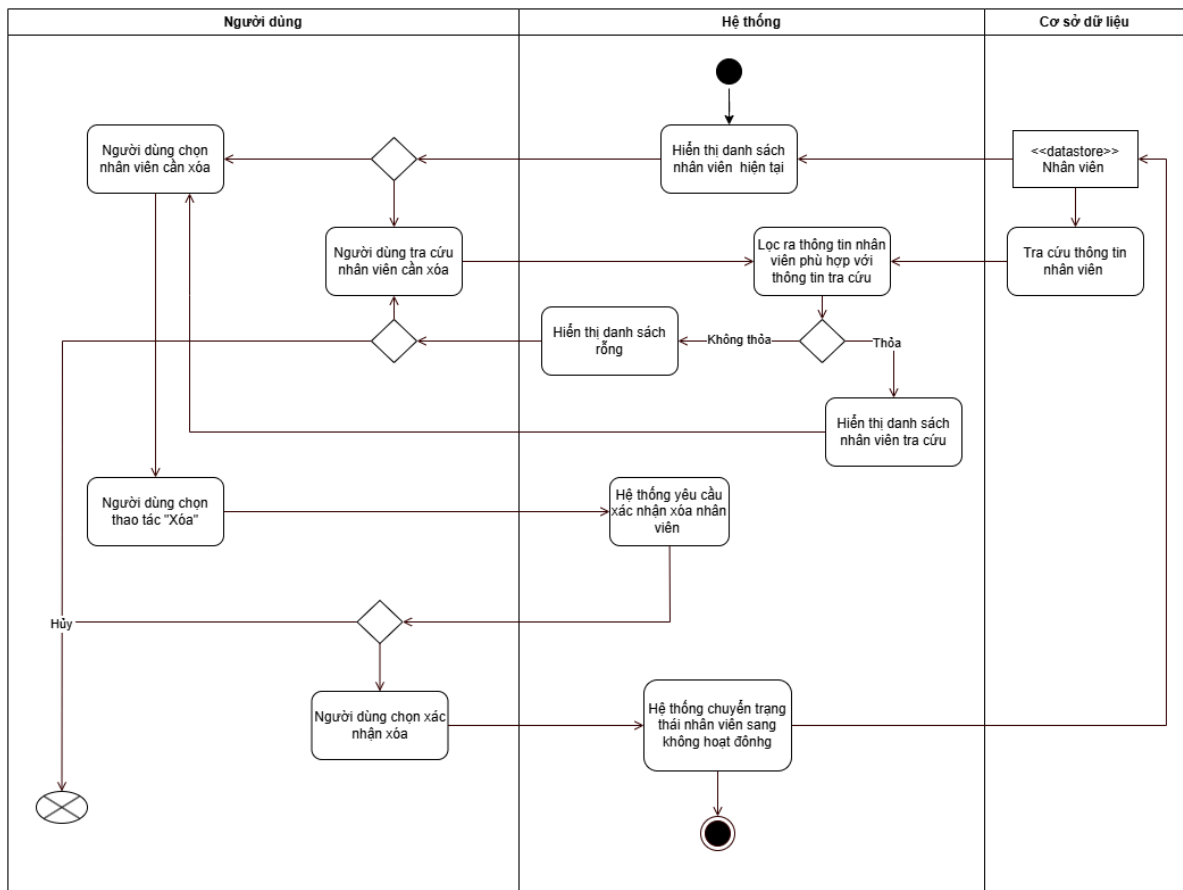
Hình 24. Activity Diagram “Xóa nhân viên”
