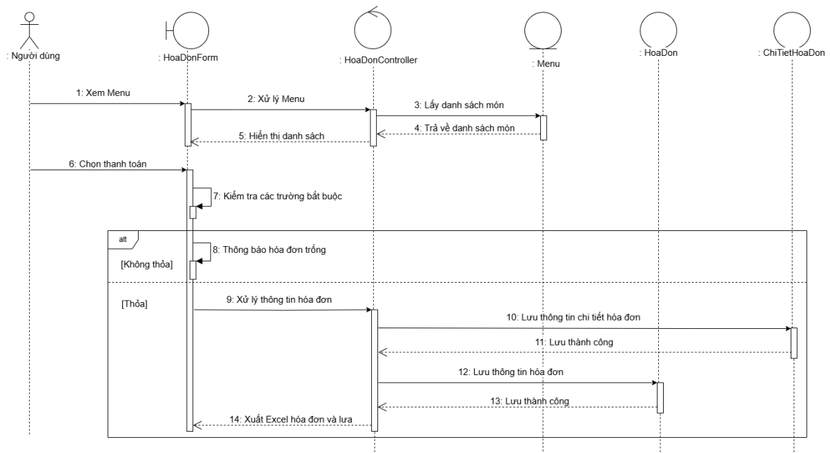
Hình 31-4. Sơ đồ tuần tự “Thanh toán” trong “Tạo hóa đơn”
