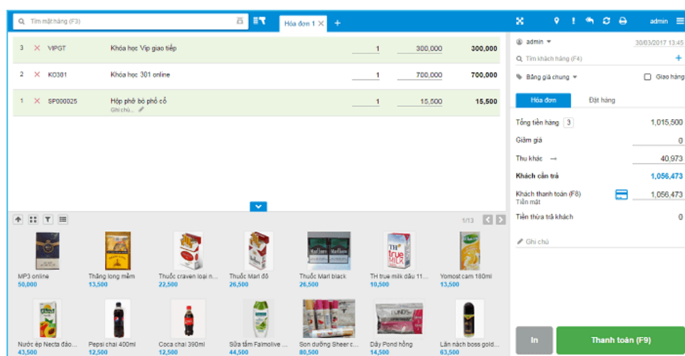
Hình 4. Hình minh họa màn hình bán hàng mới
