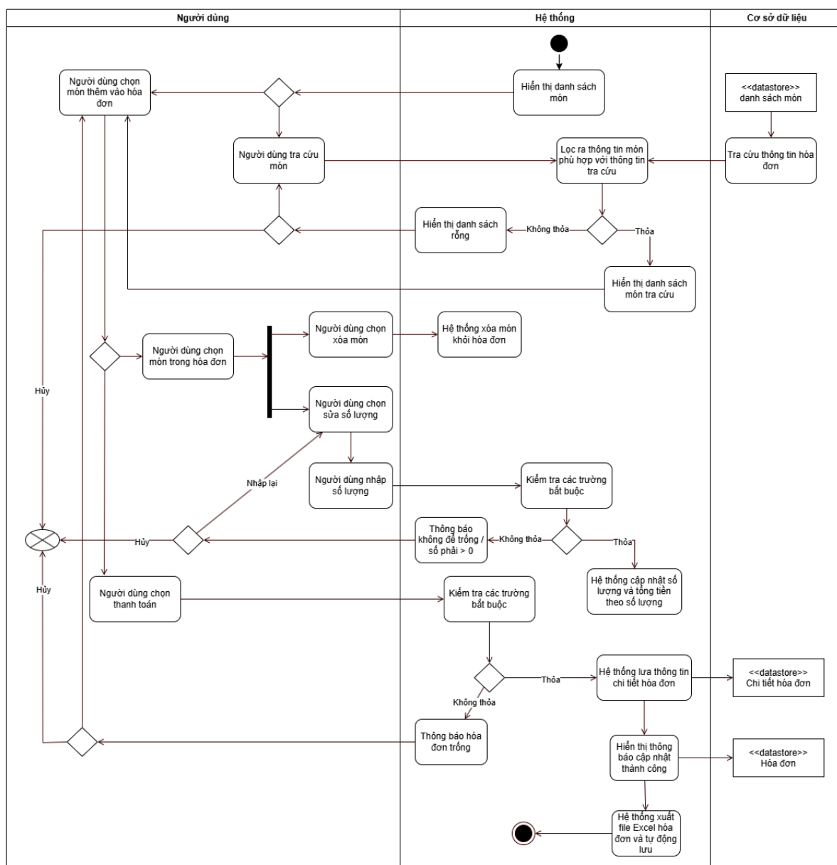
Hình 25. Activity Diagram “Tạo hóa đơn”
