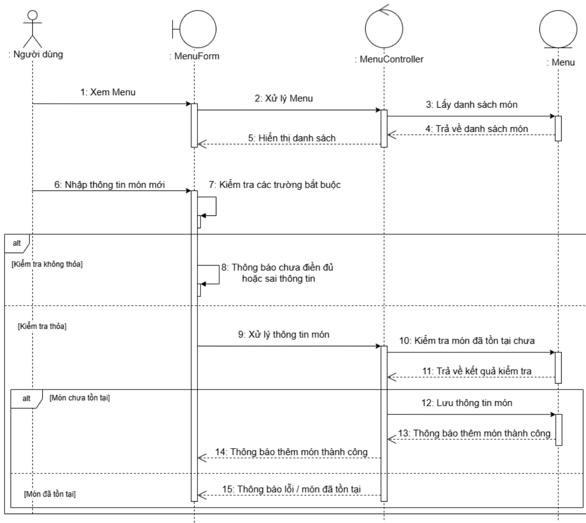
Hình 27-1. Sơ đồ tuần tự “Thêm món” trong “Quản lý Menu”
