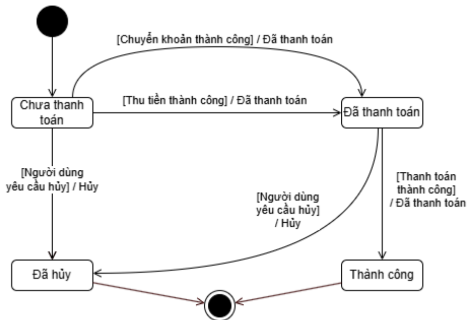
Hình 35. Sơ đồ trạng thái cho đối tượng INVOICE (hóa đơn)
