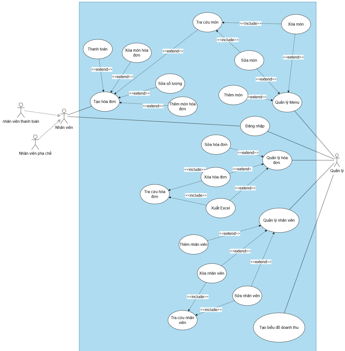
Hình 13. Sơ đồ Use-case tổng quát
