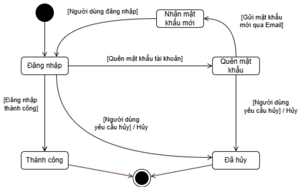
Hình 36. Sơ đồ trạng thái cho đối tượng Đăng nhập
