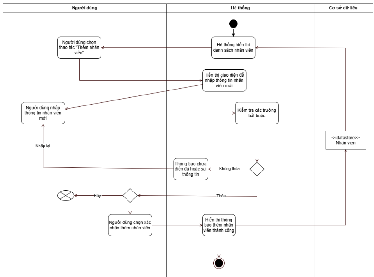
Hình 22. Activity Diagram “Thêm nhân viên”
