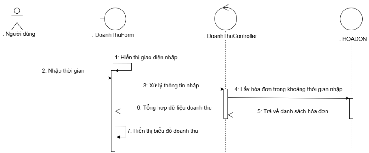
Hình 30. Sơ đồ tuần tự “Xem biểu đồ doanh thu”
