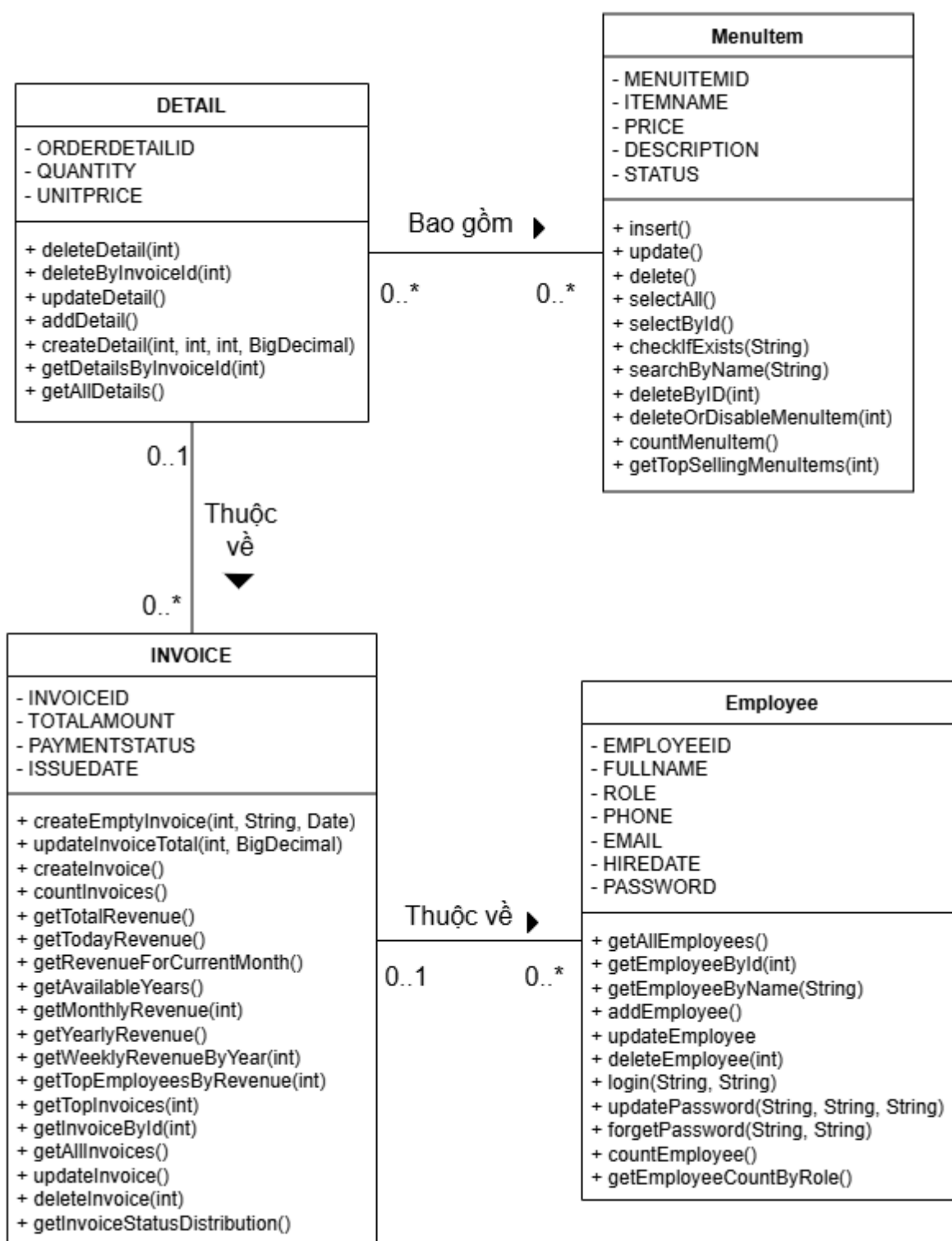
Hình 33. Sơ đồ lớp hệ thống quản lý quán Cafe mức phân tích
