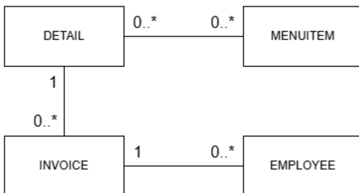
Hình 32. Sơ đồ lớp hệ thống quản lý quán Cafe
