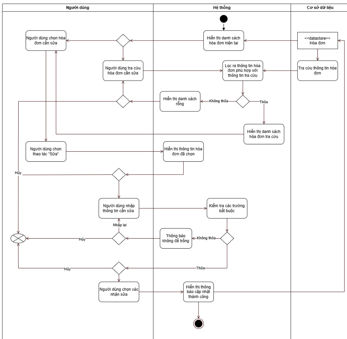
Hình 18. Activity Diagram “Sửa hóa đơn”
