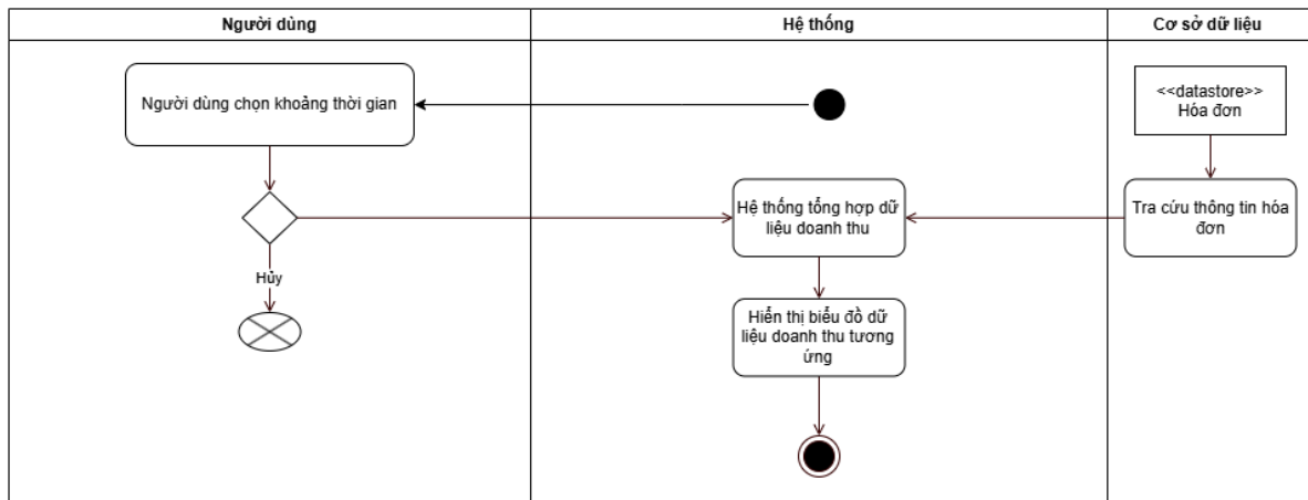
Hình 21. Activity Diagram “Xem báo cáo doanh thu”
