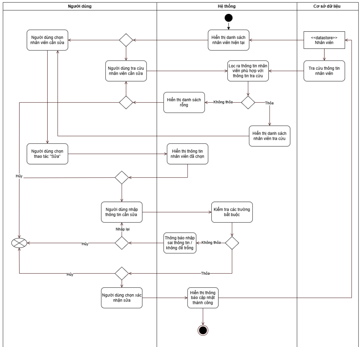
Hình 23. Activity Diagram “Sửa nhân viên”
