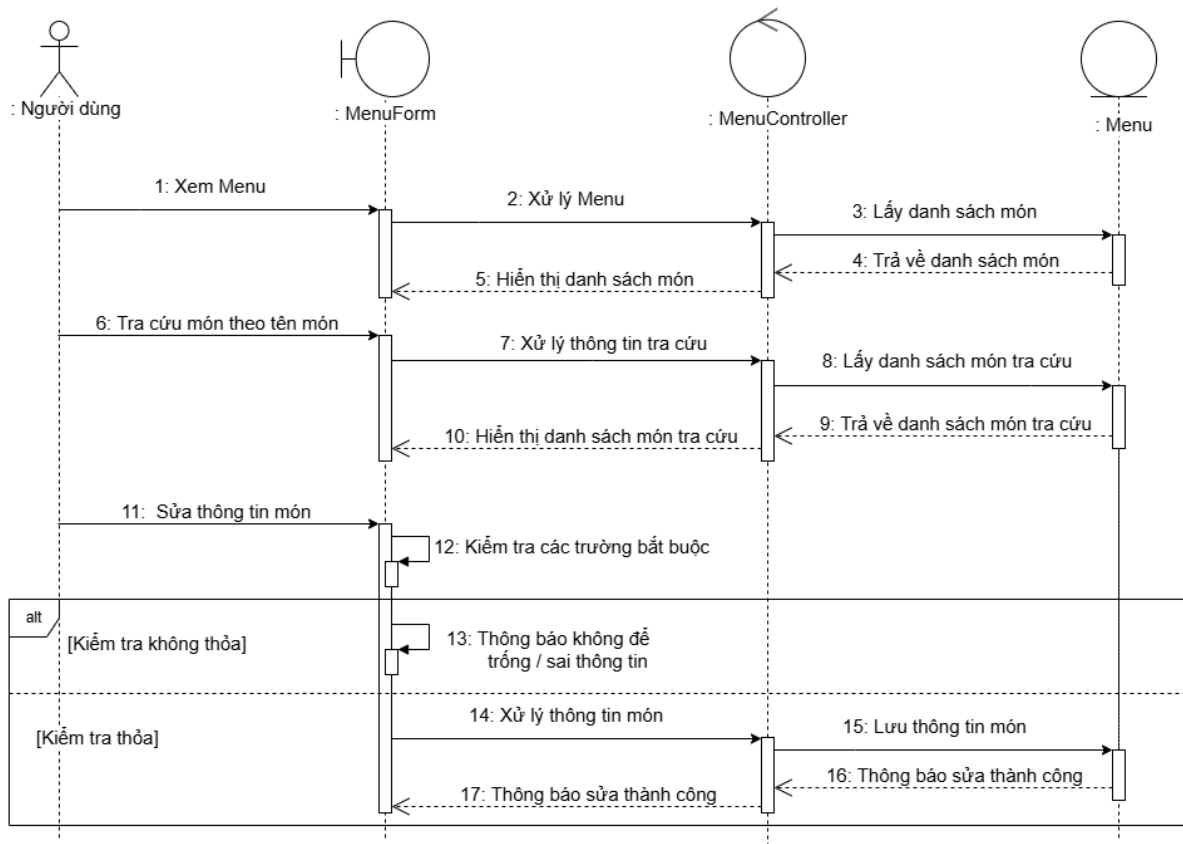
Hình 27-2. Sơ đồ tuần tự “Sửa món” trong “Quản lý Menu”
