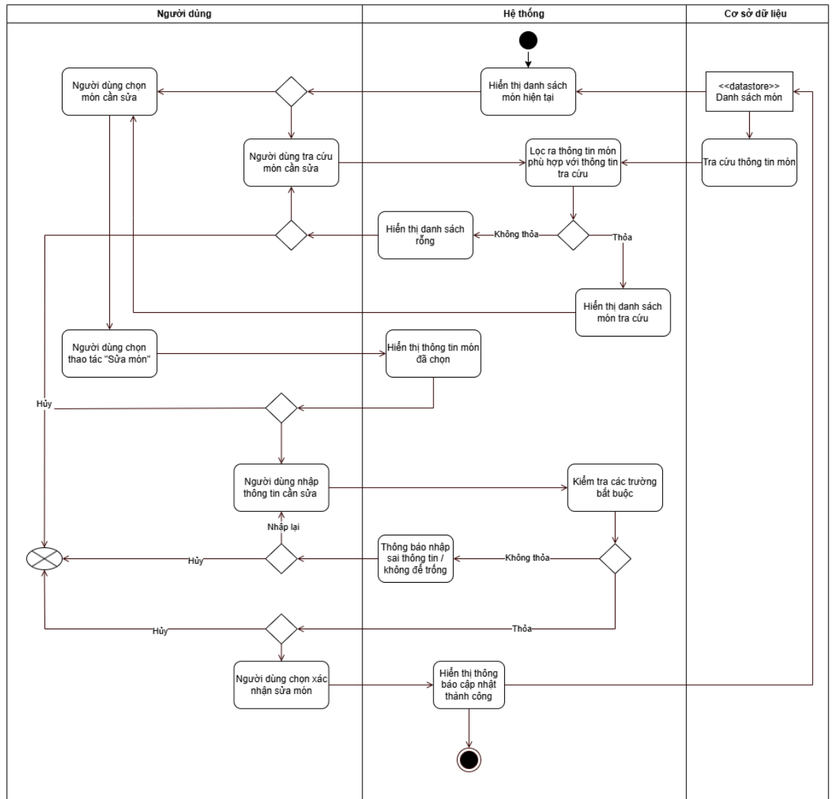
Hình 16. Activity Diagram “Sửa món”
