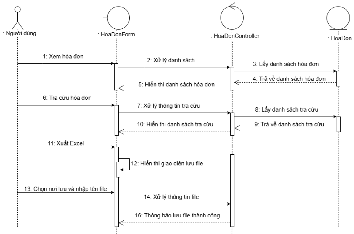
Hình 29-3. Sơ đồ tuần tự “Xuất Excel” trong “Quản lý hóa đơn”
