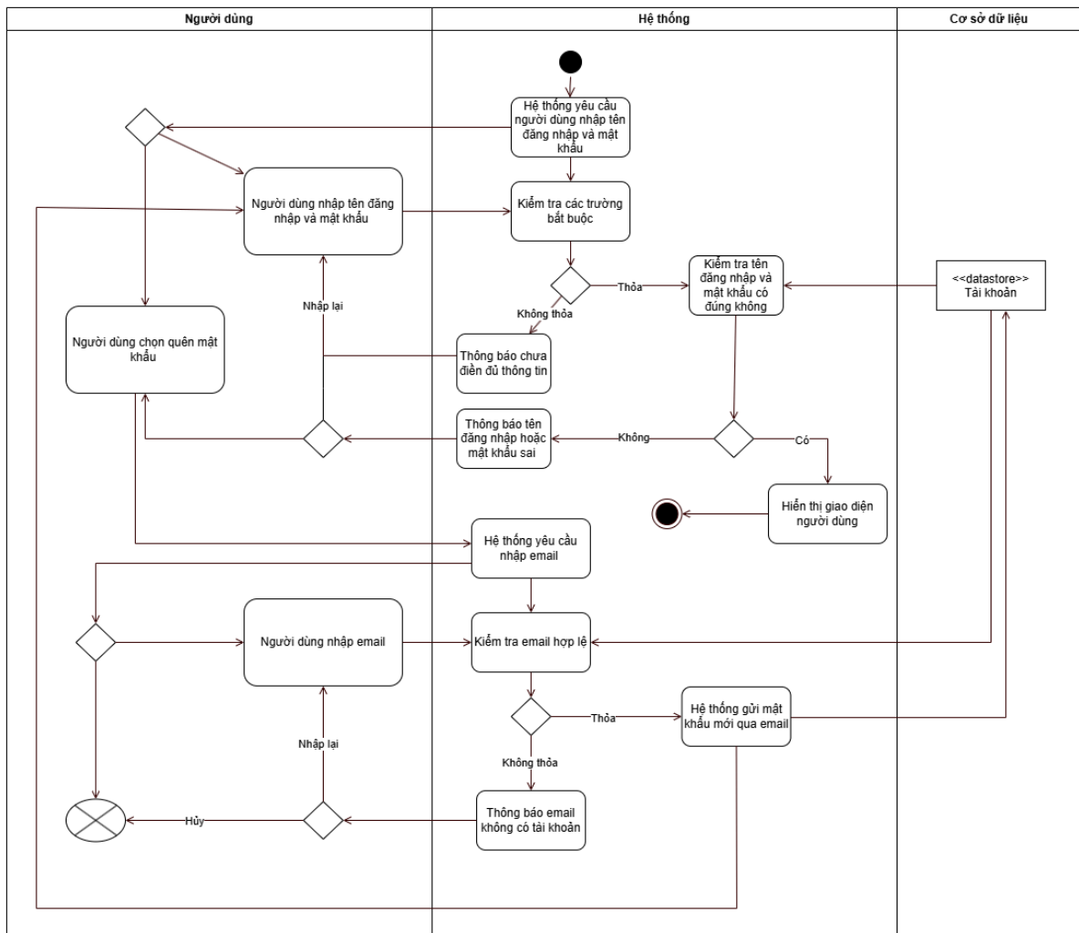
Hình 14. Activity Diagram “Đăng nhập”
