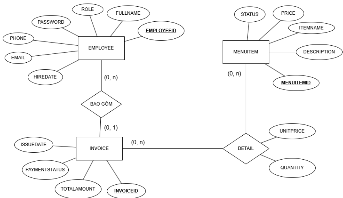
Hình 37. Mô hình dữ liệu quan hệ của hệ thống quản lý quán Cafe
