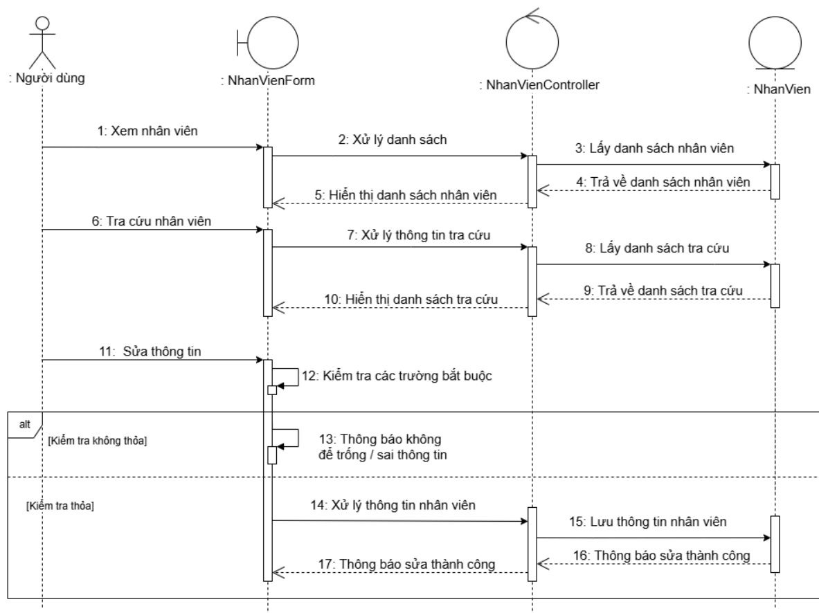
Hình 28-2. Sơ đồ tuần tự “Sửa nhân viên” trong “Quản lý nhân viên”
