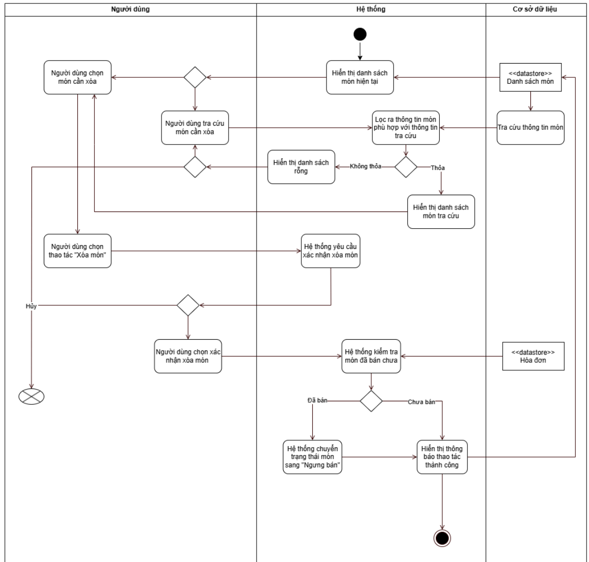
Hình 17. Activity Diagram “Xóa món”
