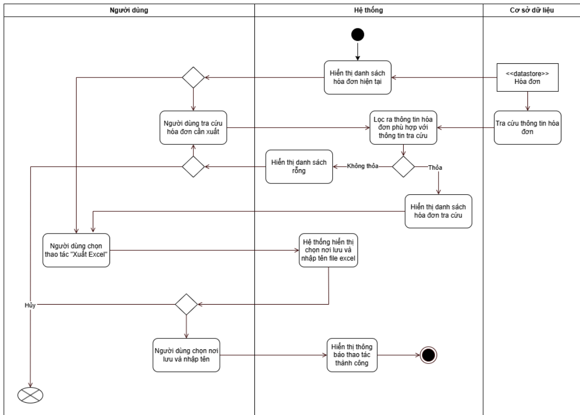
Hình 20. Activity Diagram “Xuất Excel”
