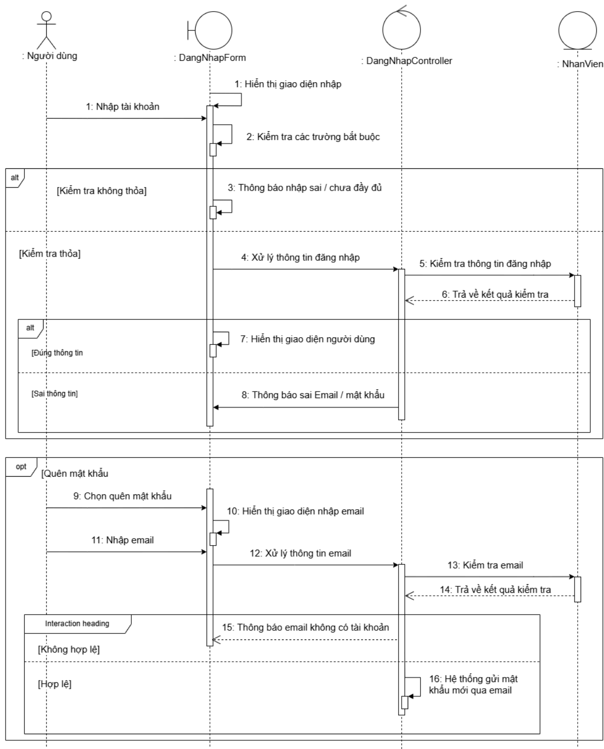
Hình 26. Sơ đồ tuần tự “Đăng nhập”
