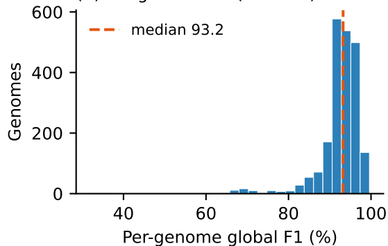
(B) Per-genome F1 (n=2151)
