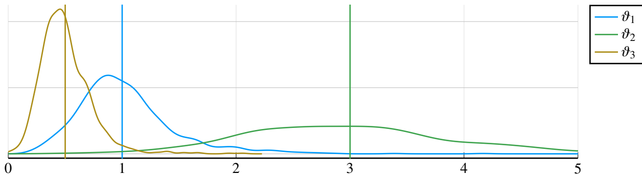
length scales \vartheta
