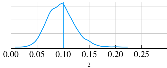
length scales \vartheta
