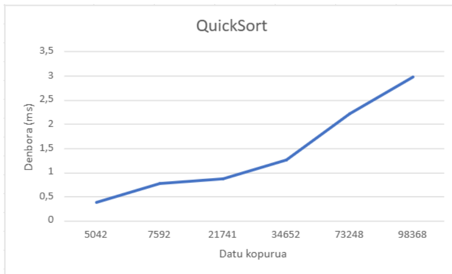
Figure 6.2: Quick Sort algoritmoaren exekuzio-denbora grafikoki
