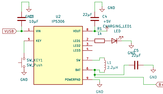
Charging IC
