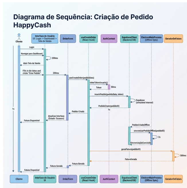
Figure 3: Diagrama de Sequência
