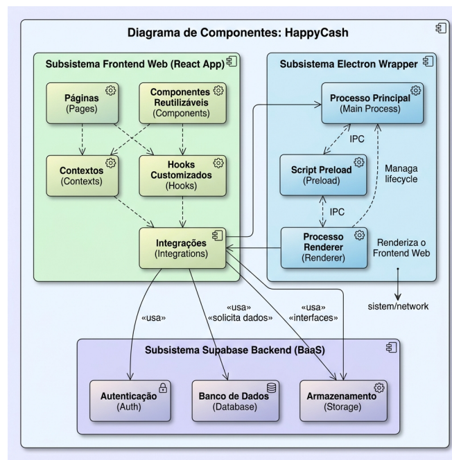
Figure 4: Diagrama de Componentes
