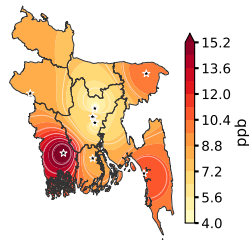
(d) \text{O}_3 surface
