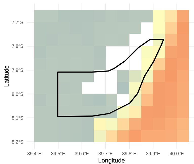
SSP5–8.5 (2080)
