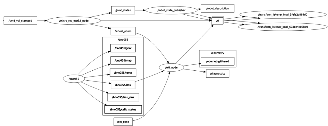
Figure 2: Systemarchitektur des Kalman-Filters in ROS2
