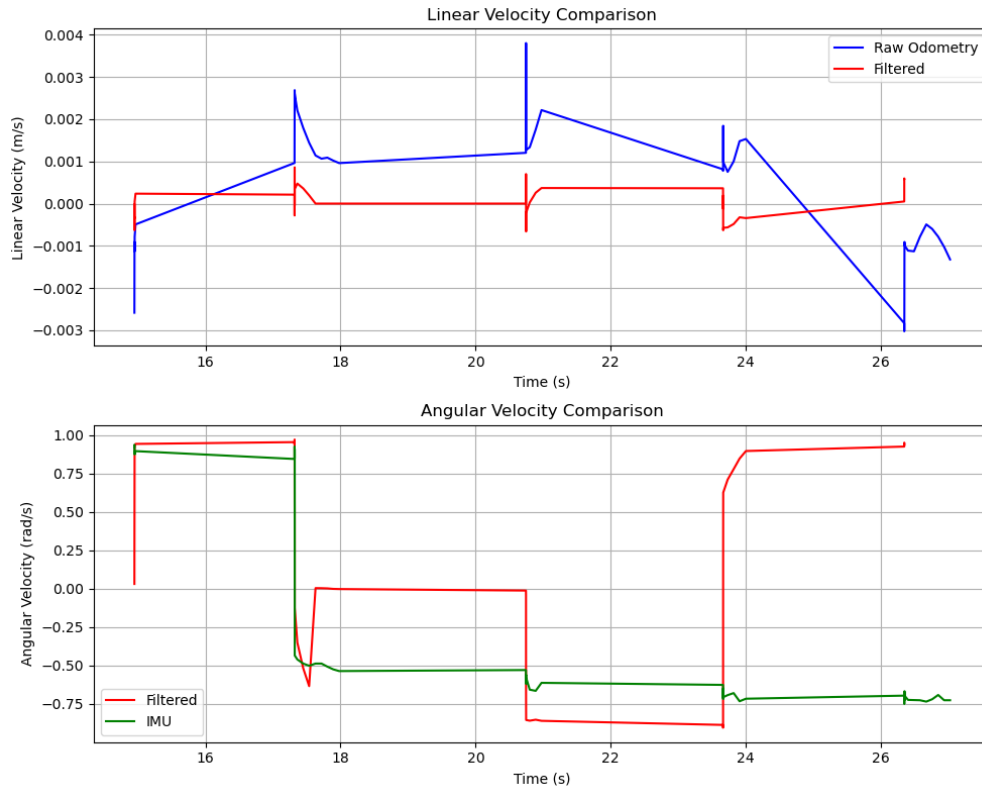
Figure 7: Vergleich der Geschwindigkeiten von Kurvenfahrt Test
