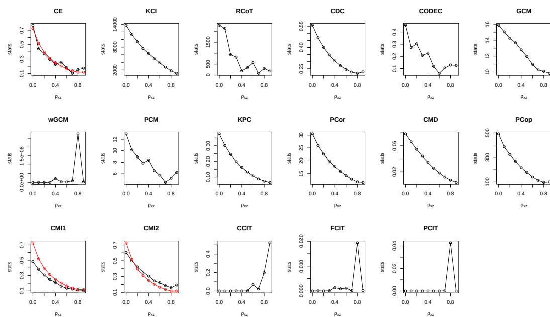
图 4.7: 在二元正态 Copula 函数上仿真条件独立性关系的评估实验结果，图中红线为真实值。
