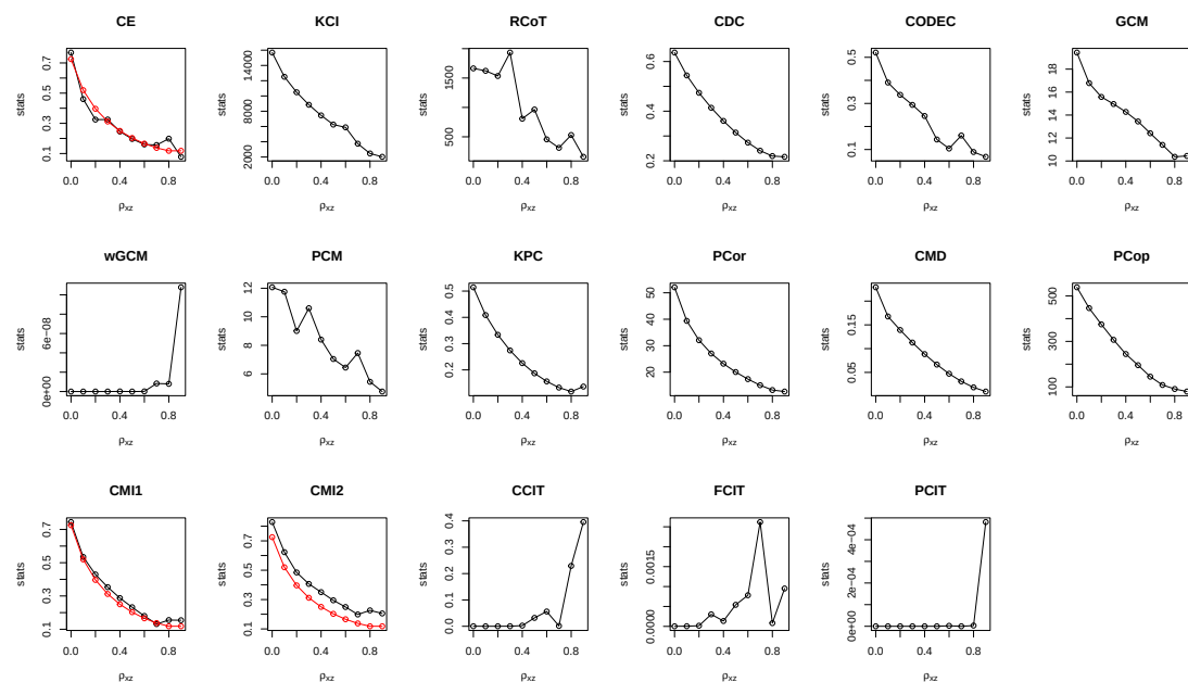
图 4.6: 在二元正态分布上仿真条件独立性关系的评估实验结果，图中红线为真实值。
