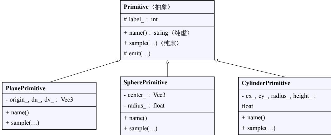
图 3 Primitive 抽象基类与派生类的 UML 类图（空心三角箭头表示继承）
