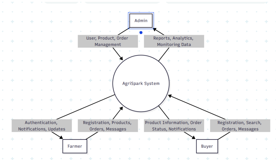
Level-0 DFD
