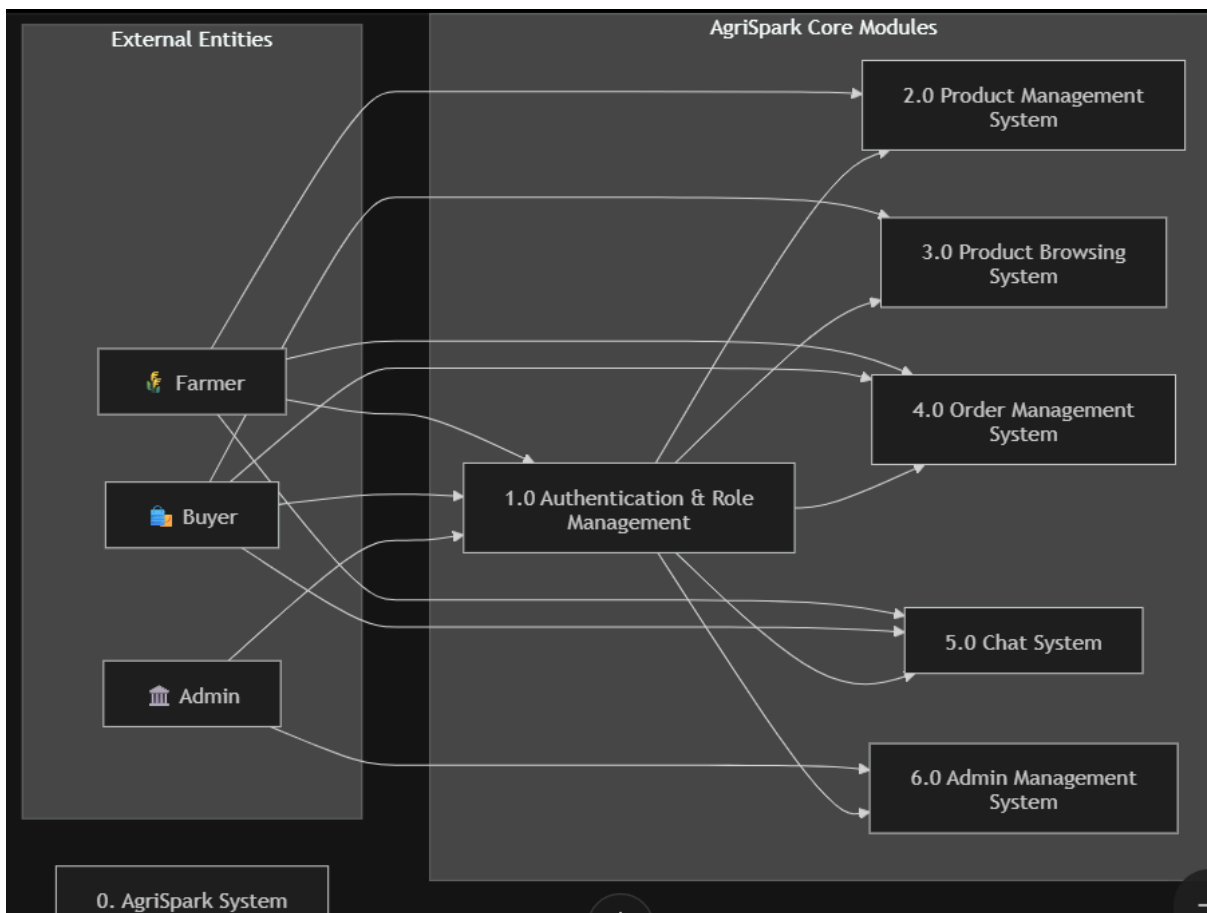
Level-0 DFD
