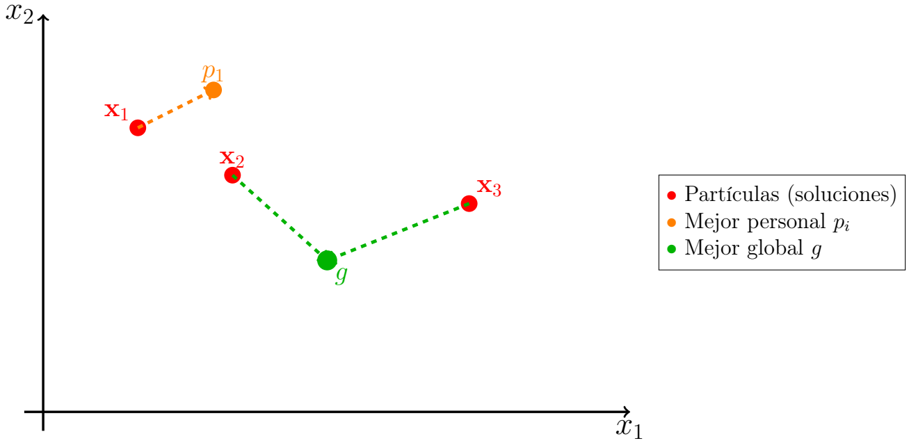
Figura 6.3: Esquema conceptual del enjambre PSO en un espacio de búsqueda bidimensional [7].
