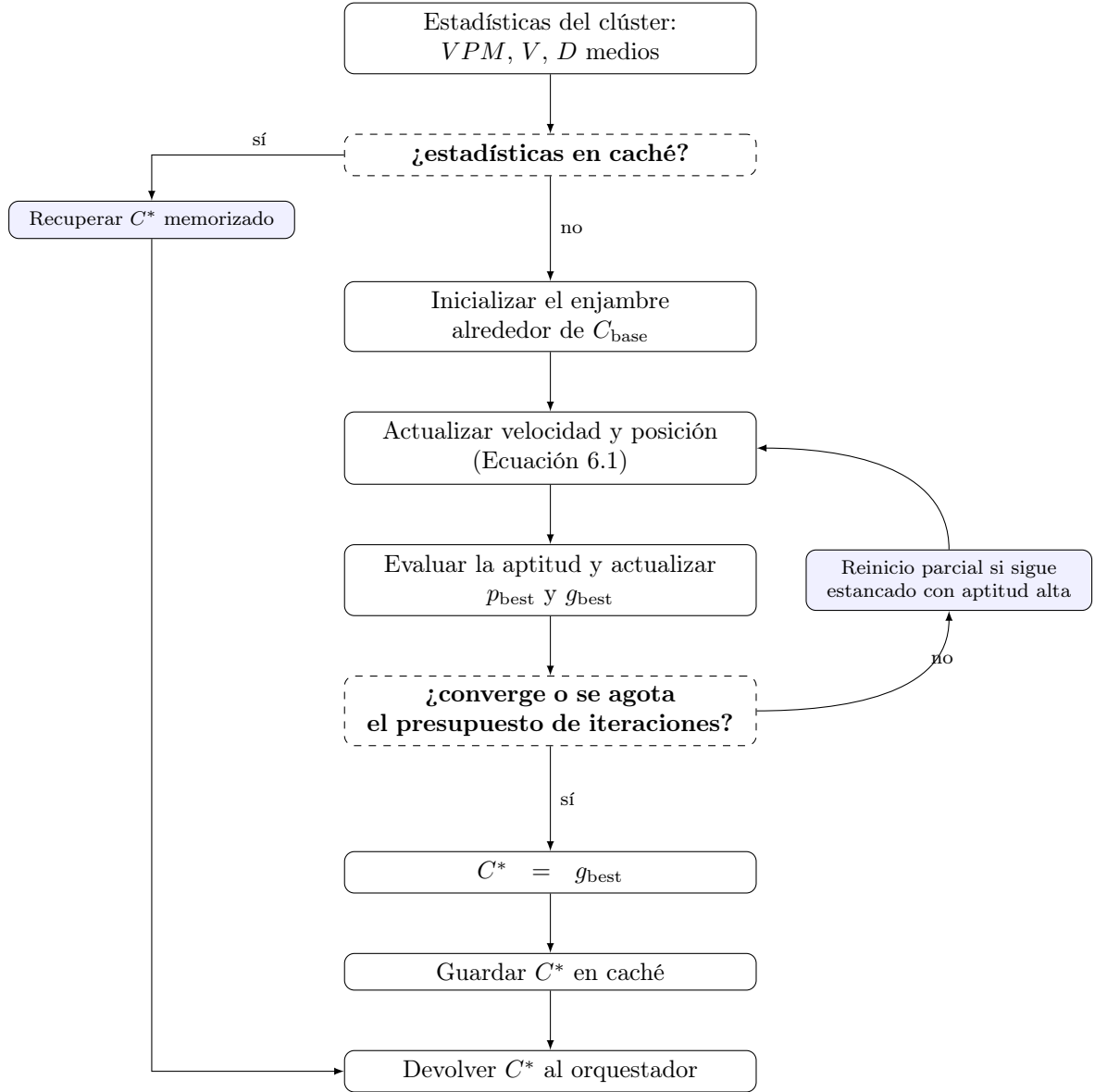
Figura 6.4: Bucle del PSO unidimensional con memoización. Un acierto de caché entrega el ciclo memorizado en menos de un milisegundo; en caso contrario se ejecuta el enjambre hasta converger o agotar su presupuesto de iteraciones. Ambas ramas confluyen en la entrega de C^* al orquestador. El tamaño del enjambre, los umbrales y la regla de reinicio figuran en la Tabla 6.4.
