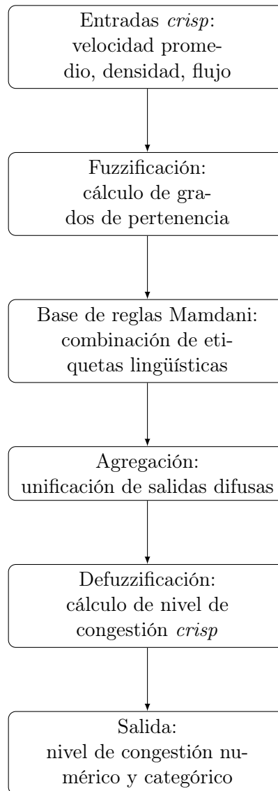
Figura 6.2: Etapas principales de un sistema de inferencia difusa tipo Mamdani aplicado a congestión vehicular [25, 53].
