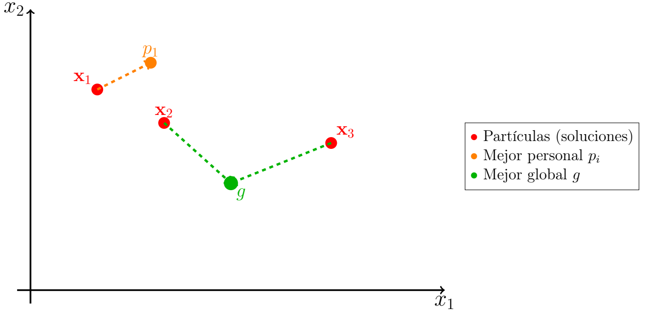
Figura 6.4: Esquema conceptual del enjambre PSO en un espacio de búsqueda bidimensional [7].
