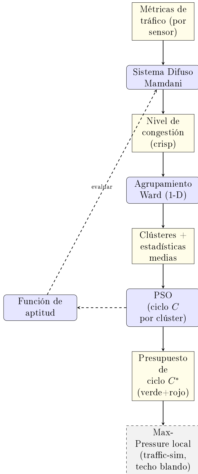
Figura 6.4: Arquitectura del módulo traffic-sync integrando lógica difusa Mamdani, agrupamiento jerárquico de Ward y optimización PSO de ciclo; la capa Max-Pressure local (fuera de traffic-sync) recibe el presupuesto de ciclo como techo blando.
