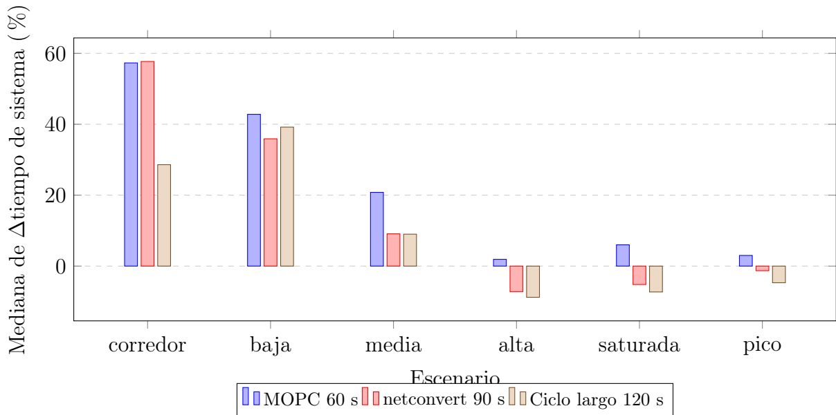
Figura 8.6: Mediana de la variación porcentual del tiempo total de sistema ( summary.xml ) del sistema propuesto respecto de cada plan fijo, por escenario. Valores negativos, presentes en demanda_alta, demanda_saturada y hora_pico frente a los planes de 90 s y 120 s, indican que el plan fijo de referencia iguala o supera al sistema propuesto en esa métrica agregada.
