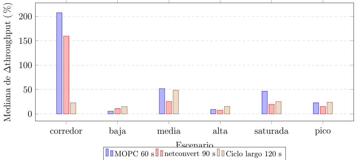
Figura 8.5: Mediana de la variación porcentual del throughput (vehículos que completan viaje) del sistema propuesto respecto de cada plan fijo, por escenario. La mediana se calcula sobre las 10 corridas de cada celda, favorables y desfavorables por igual, para evitar sesgo de selección; valores positivos indican ventaja del sistema propuesto.
