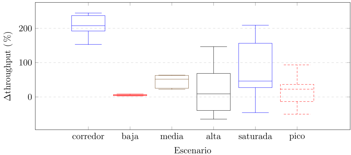
Figura 8.8: Distribución completa, por escenario, de la variación porcentual de throughput sobre las diez semillas de la campaña MOPC 60 s. La caja abarca el rango intercuartílico y la línea central la mediana; los bigotes marcan el valor observado más extremo dentro de 1,5 RIC. La dispersión es reducida en corredor y demanda_baja, donde el sistema propuesto domina en las diez semillas, y crece marcadamente en demanda_alta y demanda_saturada, donde el rango intercuartílico cruza el cero: en esas dos celdas la ventaja o desventaja del sistema propuesto es sensible a la semilla concreta, reflejo del régimen de colapsos autoinducidos cerca de la capacidad de la red descrito en la Sección 8.4.9.
