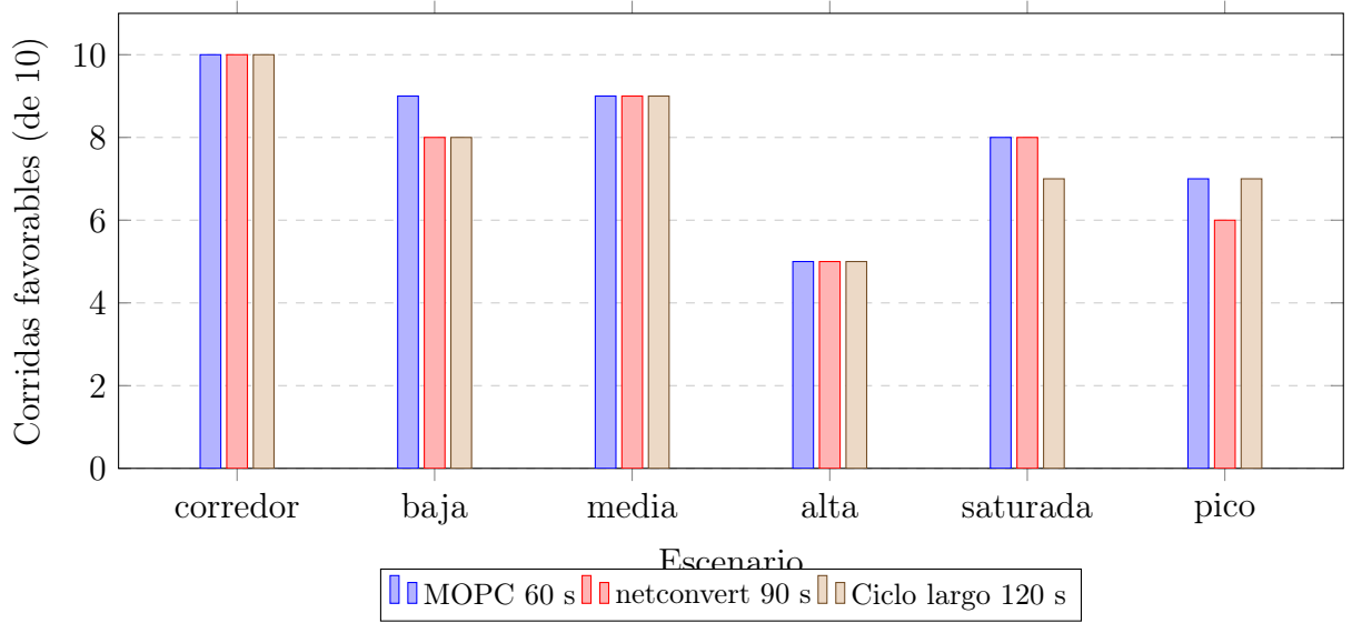
Figura 8.4: Número de corridas favorables al sistema propuesto (de 10 semillas) por escenario de demanda y campaña de comparación. Cada barra agrupa las tres campañas frente a un mismo escenario; valores cercanos a 10 indican dominancia consistente del sistema propuesto sobre el plan fijo correspondiente, independientemente de la semilla.
