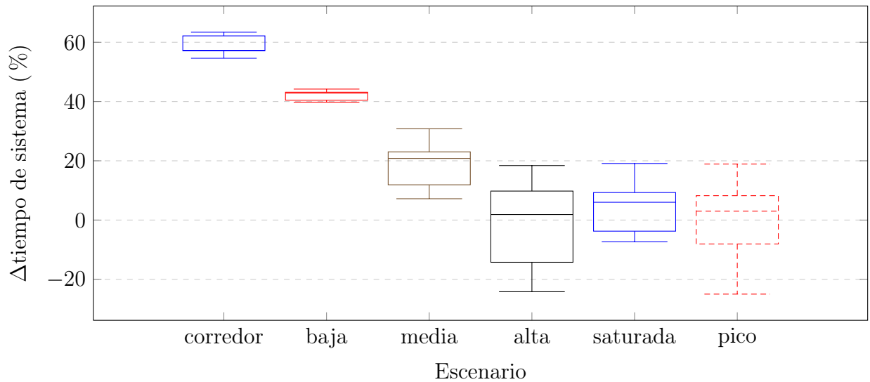
Figura 8.9: Distribución completa, por escenario, de la variación porcentual del tiempo total de sistema sobre las diez semillas de la campaña MOPC 60 s, con la misma convención de caja y bigotes que la Figura 8.8. La dispersión de esta métrica es sistemáticamente menor que la del throughput en todos los escenarios, consistente con su carácter de variable agregada continua frente al carácter más discreto y sensible al colapso del throughput; aun así, demanda_alta y hora_pico muestran cajas que cruzan el cero, confirmando que esos dos escenarios son los de resultado menos predecible entre semillas.
