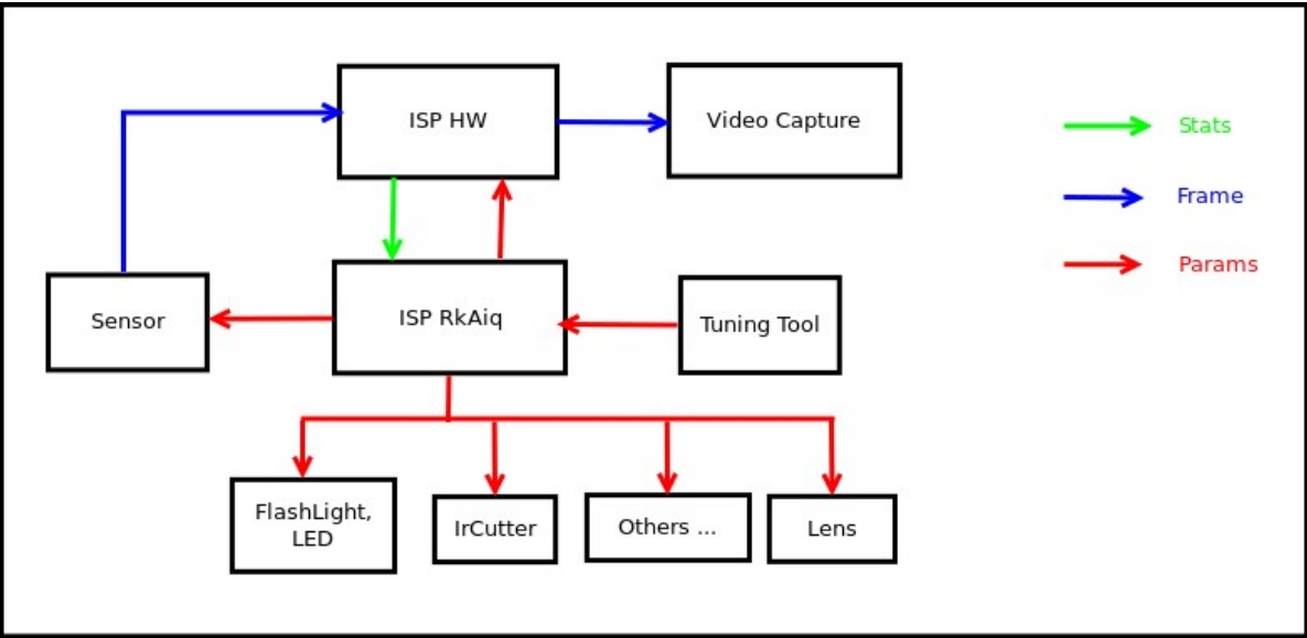
图1-1 AIQ 系统框图
