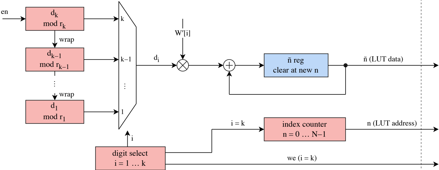
digit inverter
