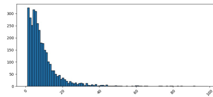
Rysunek 4.8: Przykład analizy długości tekstu z Alpha
