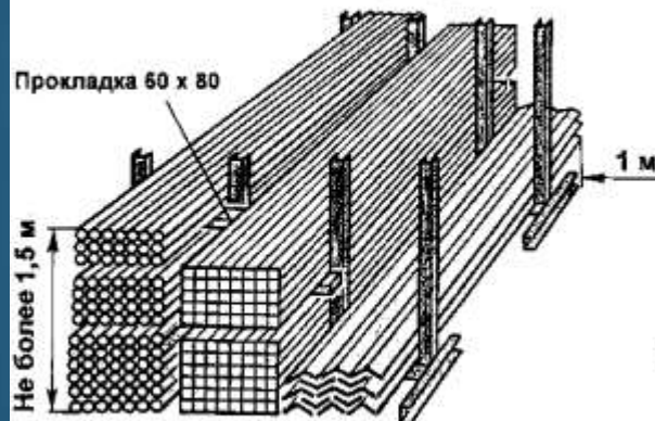
МЕЛКОСОРТНЫЙ МЕТАЛЛ В СТЕЛЛАЖАХ
