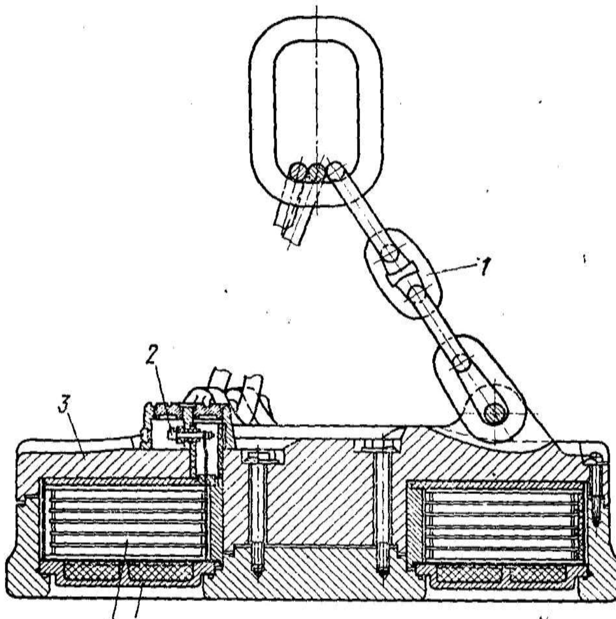
Подъемный электромагнит типа М
