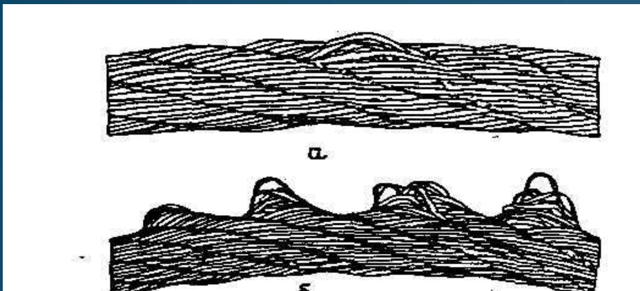
Выдавливание проволок прядей: а — в одной пряди; б — в нескольких прядях
