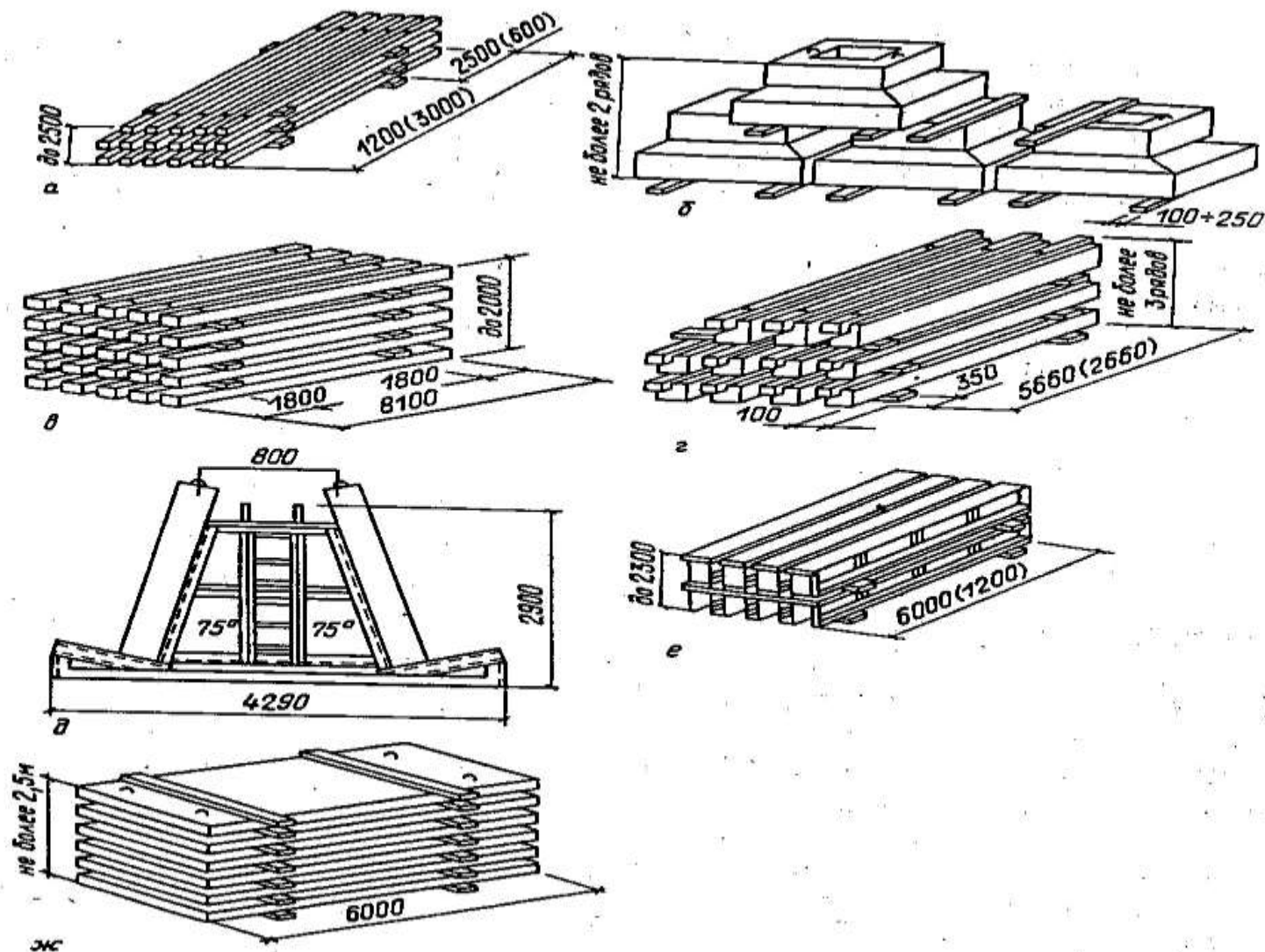
Схемы складирования конструкций на приобъектном складе: а — сваи; б — фундаментные блоки; в — колонны; г — ригели; д — панели; е — балки подкрановые; ж — плиты перекрытия
