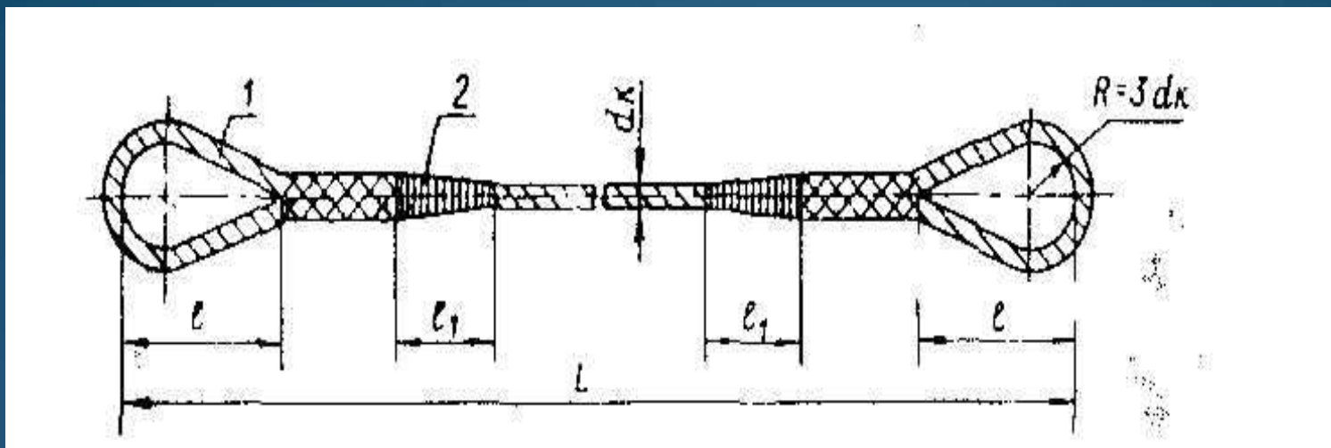
Универсальный строп, исполнение 1: 1—канат грузовой, 2—место заделки концов каната
