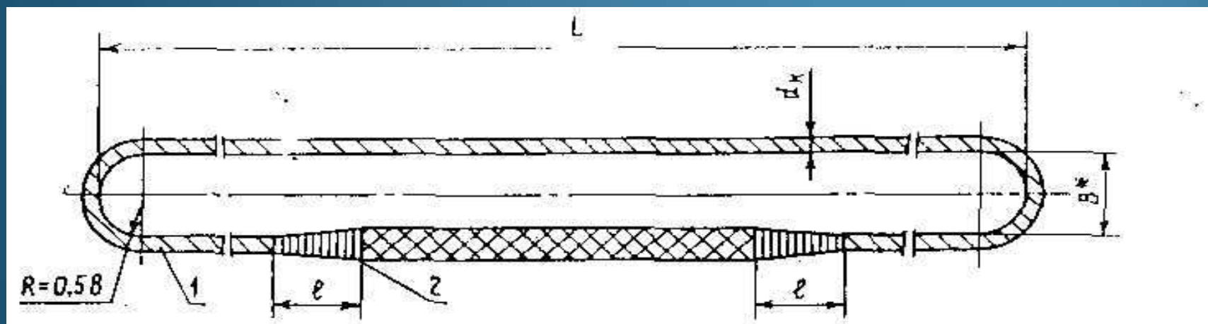
Универсальный строп, исполнение 1: 1—канат грузовой, 2—место заделки концов каната
