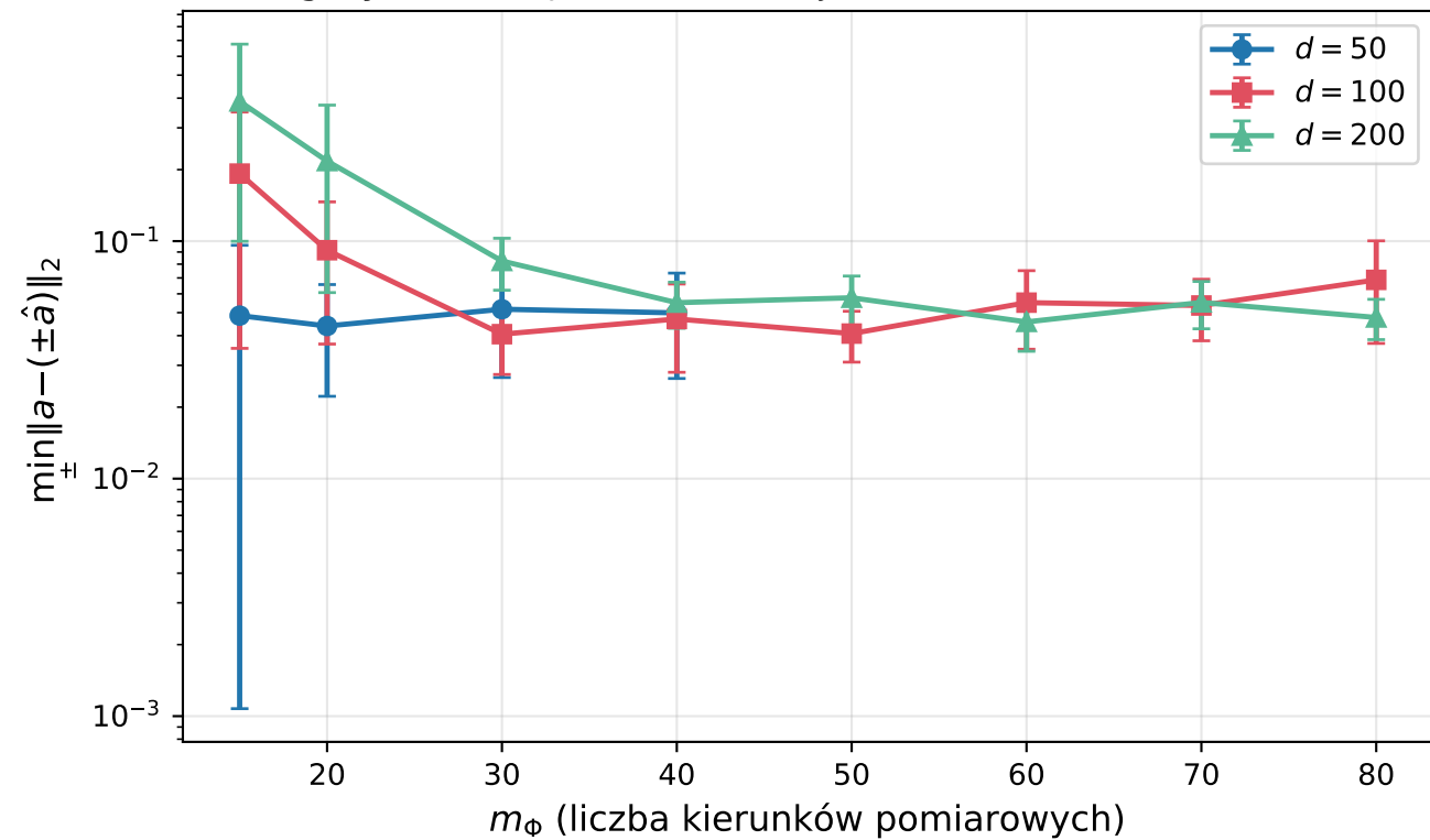
Algorytm 1: błąd rekonstrukcji wektora a ( k = 1 , m_X = 30 )
