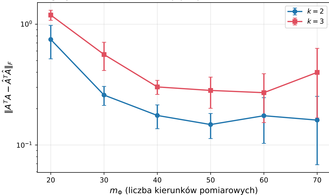
Algorytm 2: błąd rekonstrukcji podprzestrzeni ( d = 80, m_X = 40 )
