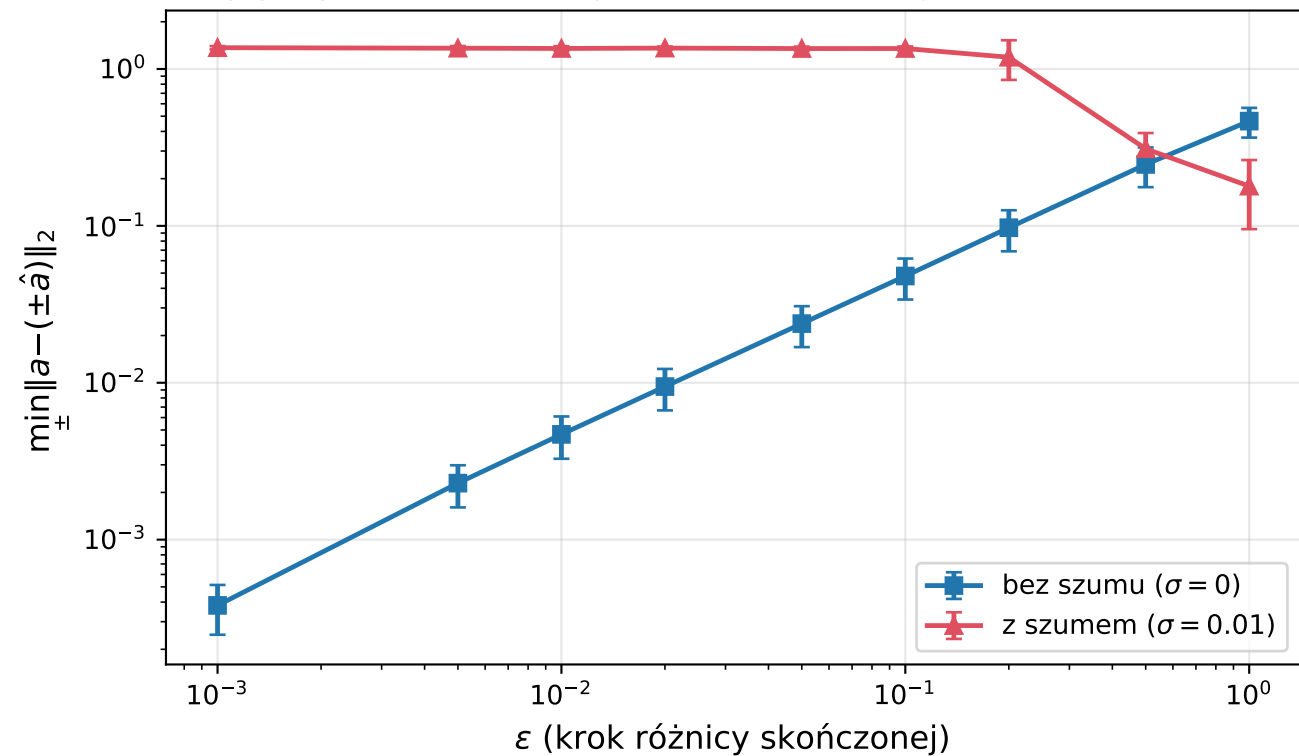
Wpływ parametru \varepsilon na jakość rekonstrukcji ( d = 100 , m_\phi = 50 )
