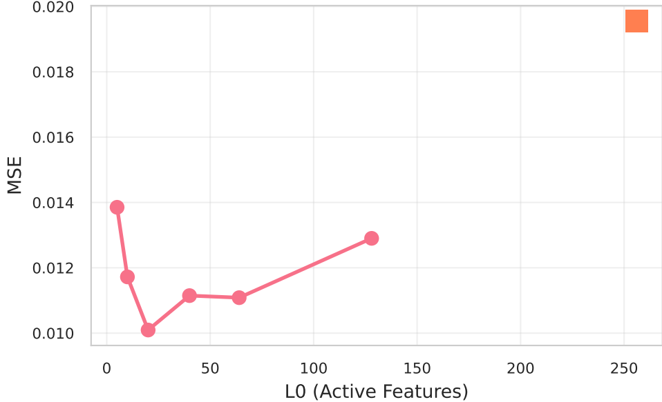
LFW: Interpretability
