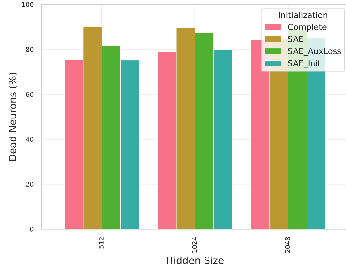
LFW Dataset
