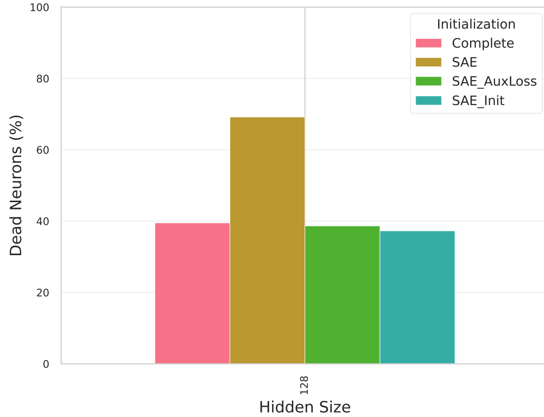
MNIST Dataset
