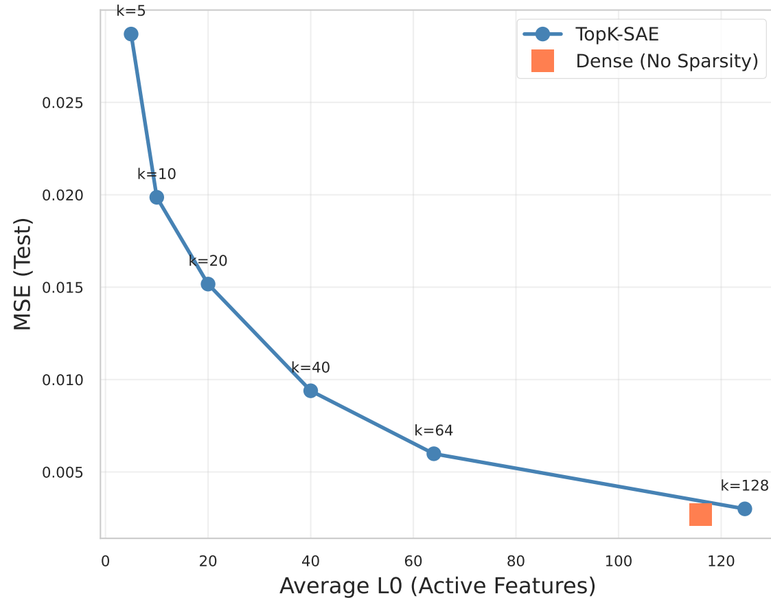
MNIST
