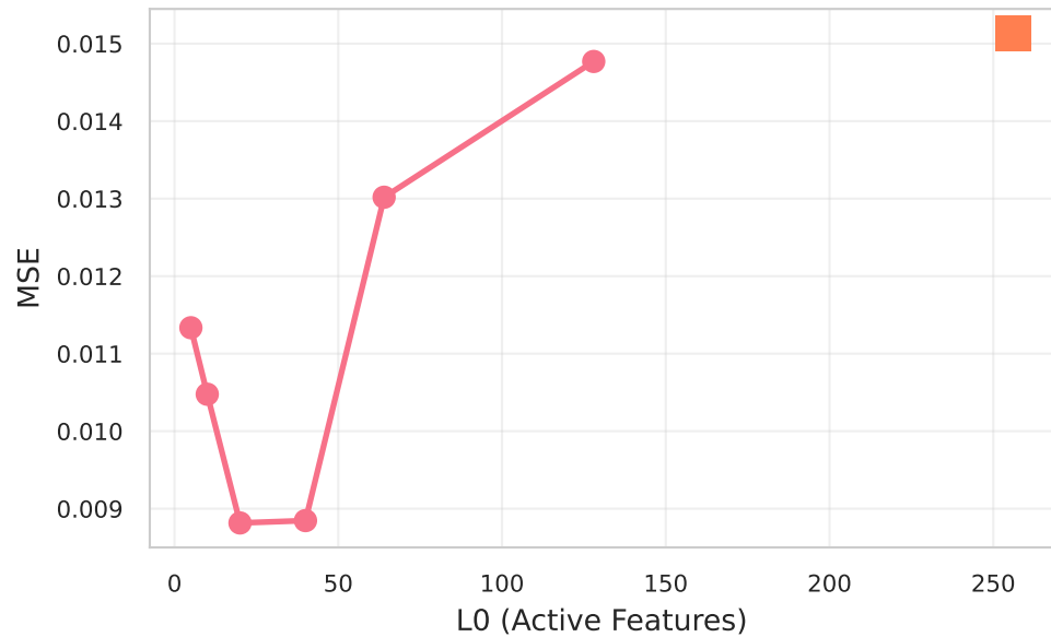
OLIVETTI: Interpretability
