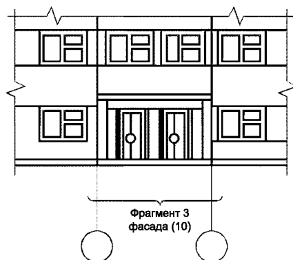
Рисунок 16 - Пример указания места размещения вынесенного фрагмента фасада
