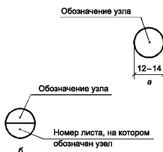
Рисунок 14 - Примеры указания обозначения узла над его изображением
