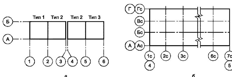
Рисунок 4 - Примеры присвоения обозначений и размещения координационных осей
