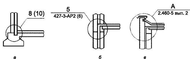
Рисунок 13 - Примеры указания мест расположения узла на плане, фасаде или разрезе
