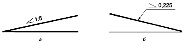
Рисунок 9 - Примеры обозначения уклона
