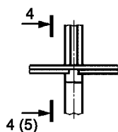
Рисунок 12 - Пример указания на чертеже секущей плоскости сечения
