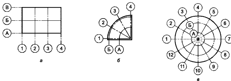
Рисунок 1 - Примеры обозначений координационных осей
