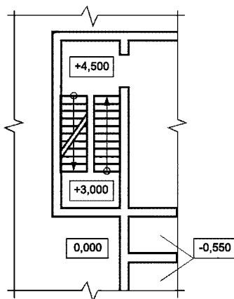
Рисунок 7 - Примеры размещения отметок на планах
