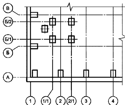
Рисунок 2 - Примеры нанесения и расположения дополнительных осей
