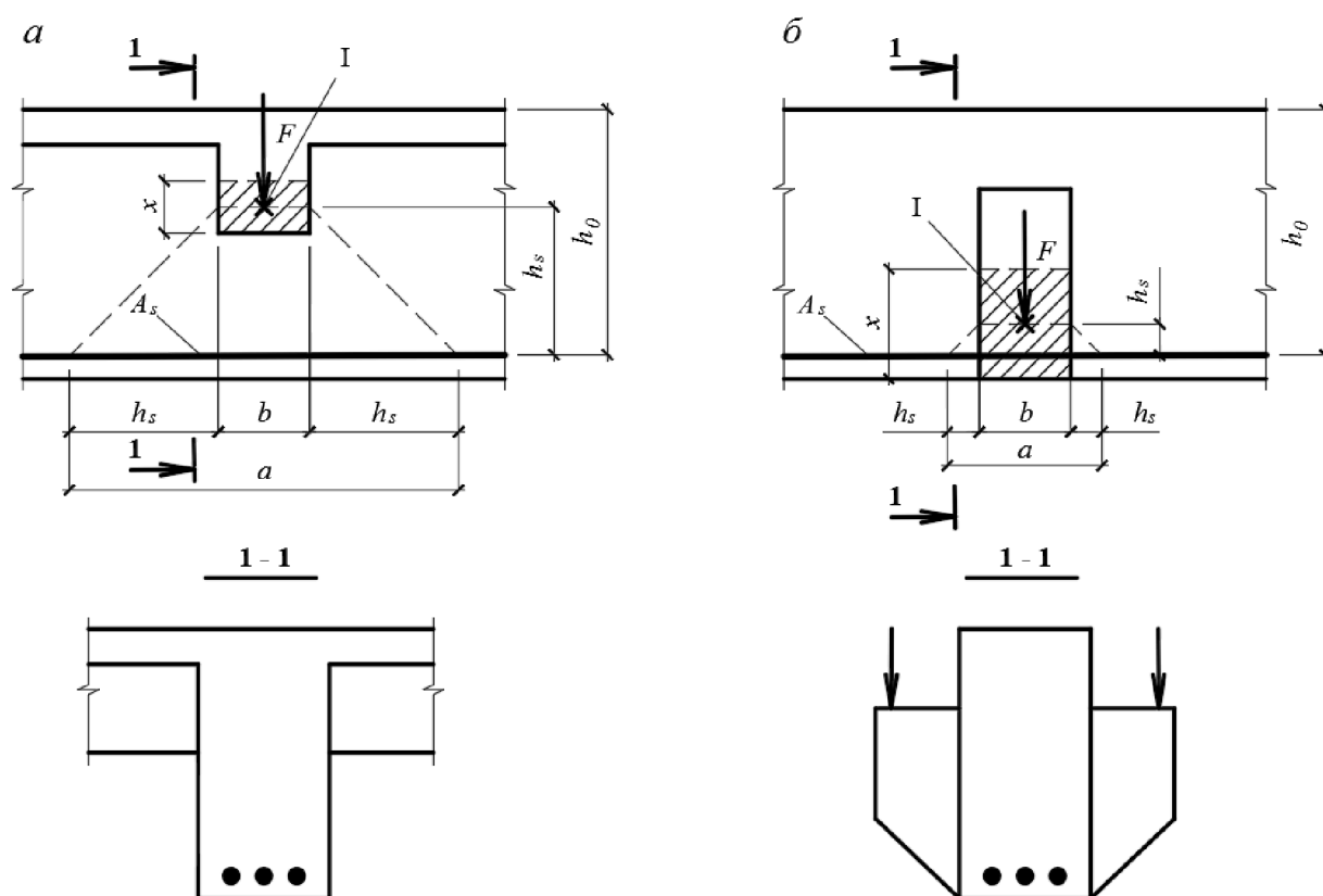
a – при примыкании балок; б – при примыкании консолей; I – центр тяжести сжатой зоны примыкающего элемента
