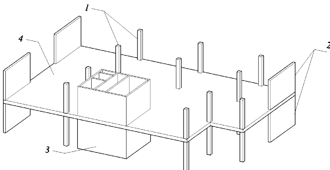
1 – колонны; 2 – стены; 3 – ядро жесткости; 4 – плита перекрытия
