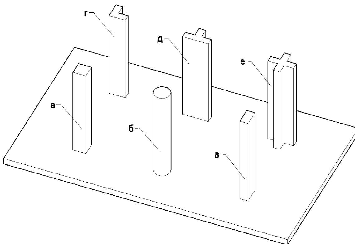
а – квадратное; б – круглое; в – прямоугольное; г – Г-образное (угловое); д – Т-образное (тавровое); е – крестообразное
